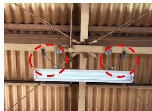
照明器具の耐震化 (武道場照明器具の振れ止め補強)
