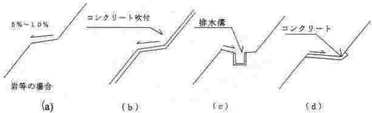
小段の横断勾配（概略図）
