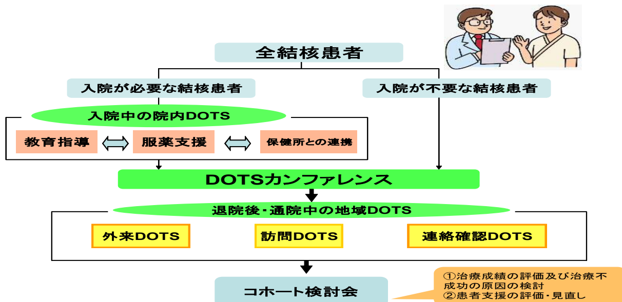
【図表3-3-14】 DOTS推進体系図
