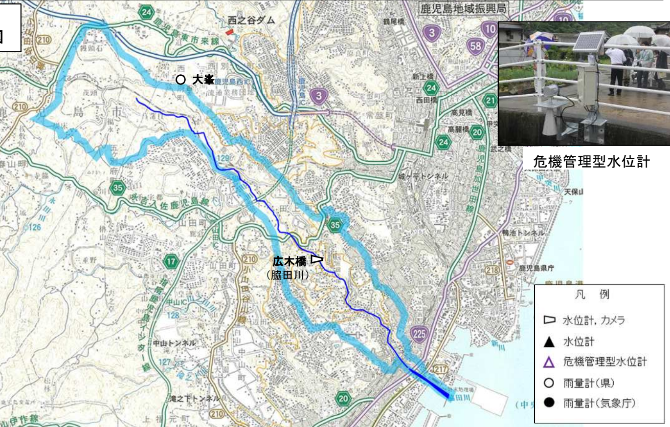
脇田川流域における 水位計・監視カメラ・雨量計の位置図
