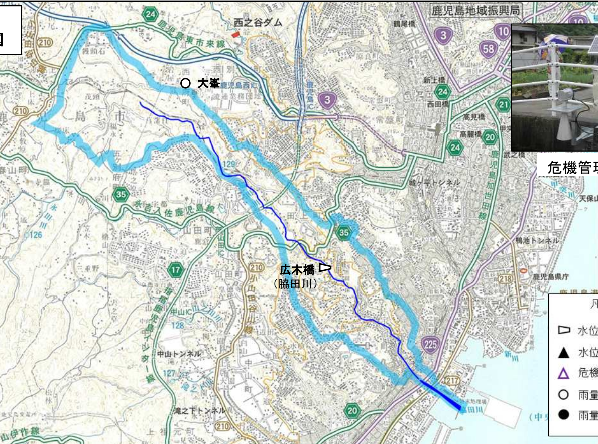
脇田川流域における 水位計・監視カメラ・雨量計の位置図
