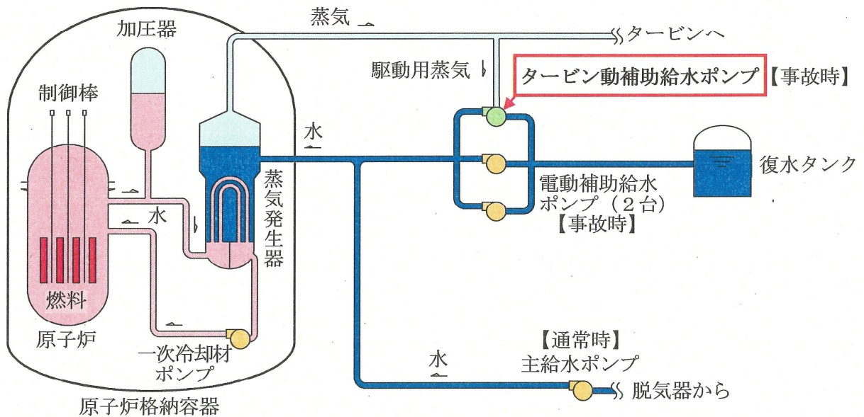
【川内原子力発電所 概略系統図】
