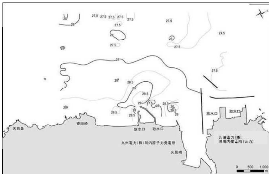
図10-4 3m層水温水平分布 (上げ潮時) 単位:℃
