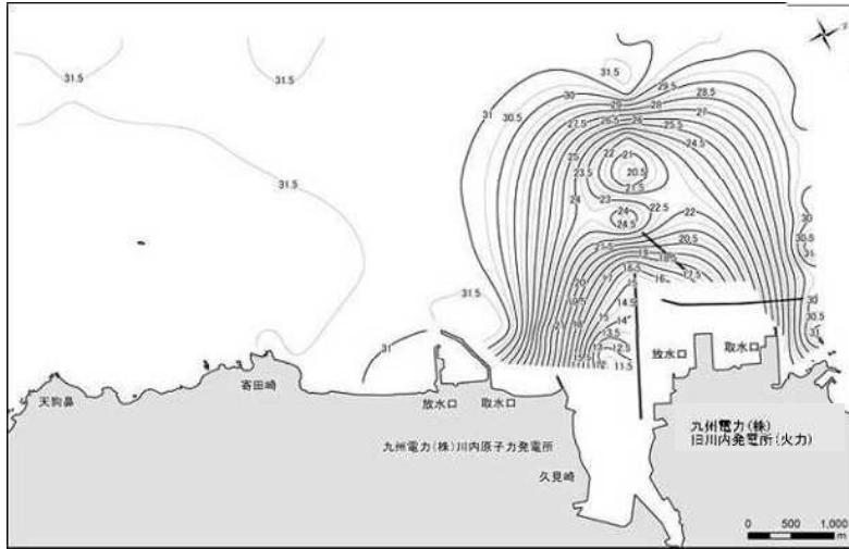
図11-1 表層(0.3m深)塩分水平分布(下げ潮時)
