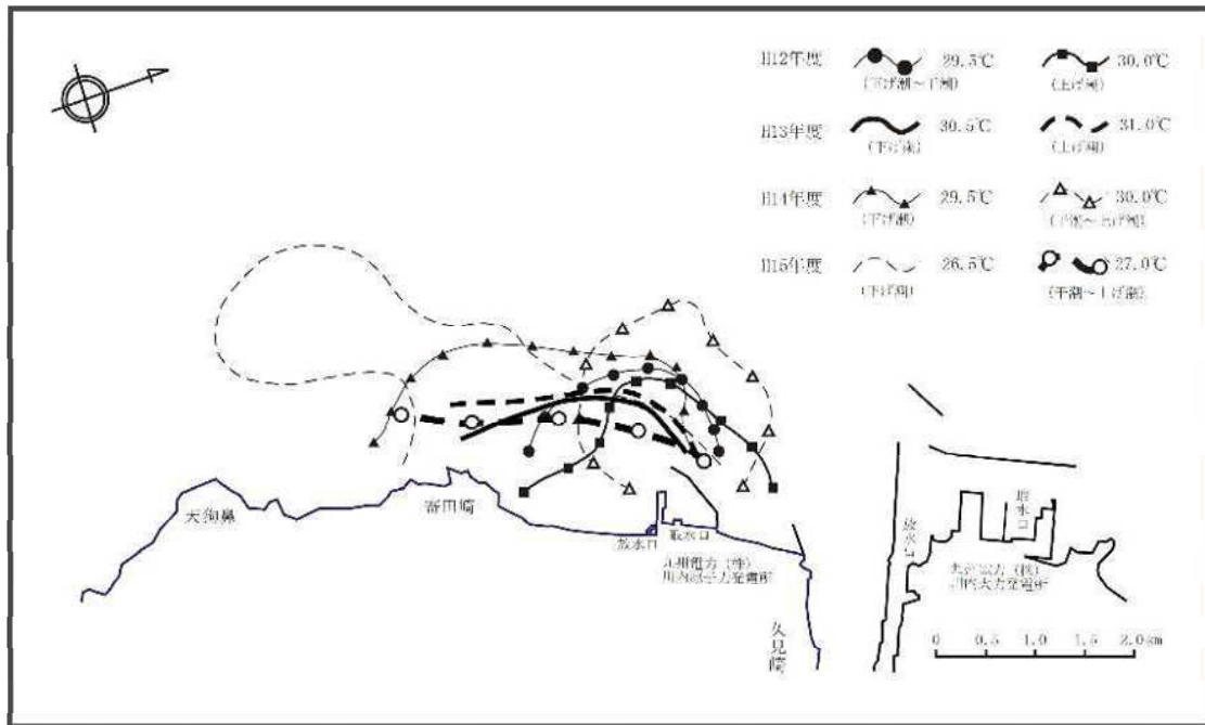
图12-5 平成12年度～15年度夏季表層(0.3m深)温排水拡散範圍
