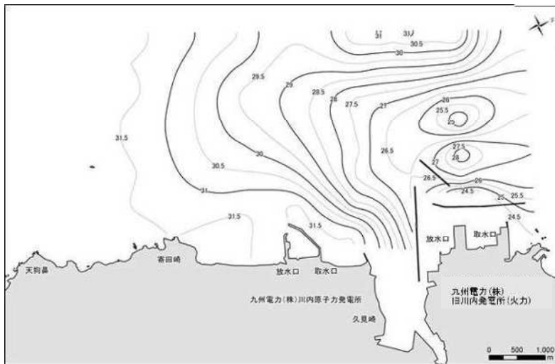
図11-2 表層(0.3m深)塩分水平分布(上げ潮時)
