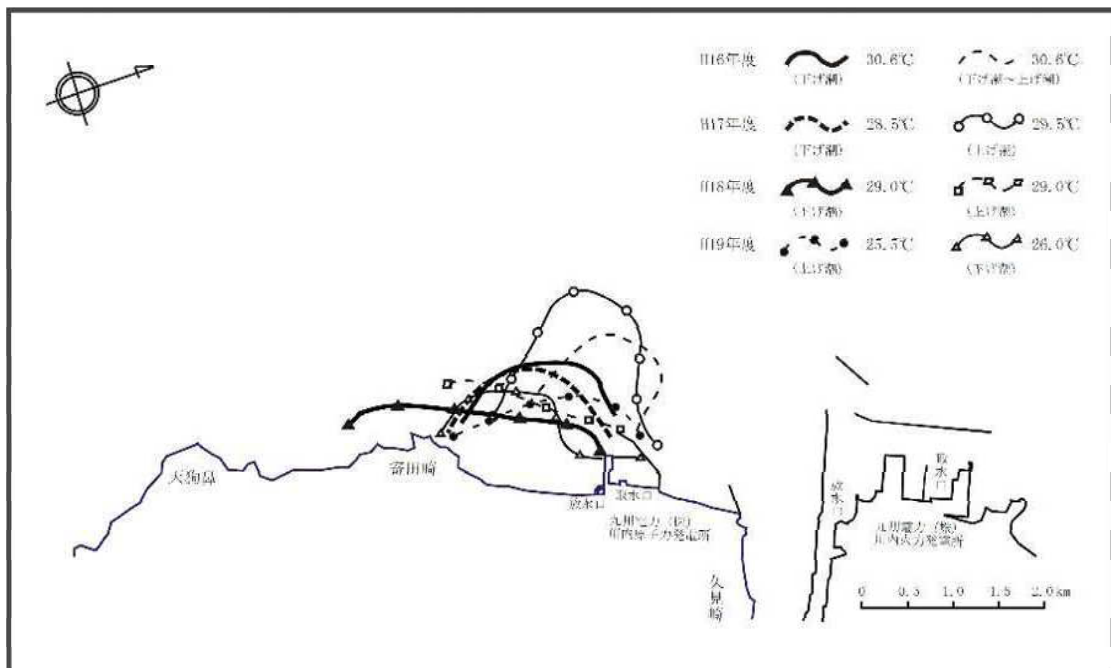
图12-6 平成16年度～19年度夏季表層(0.3m深)温排水拡散範圍
