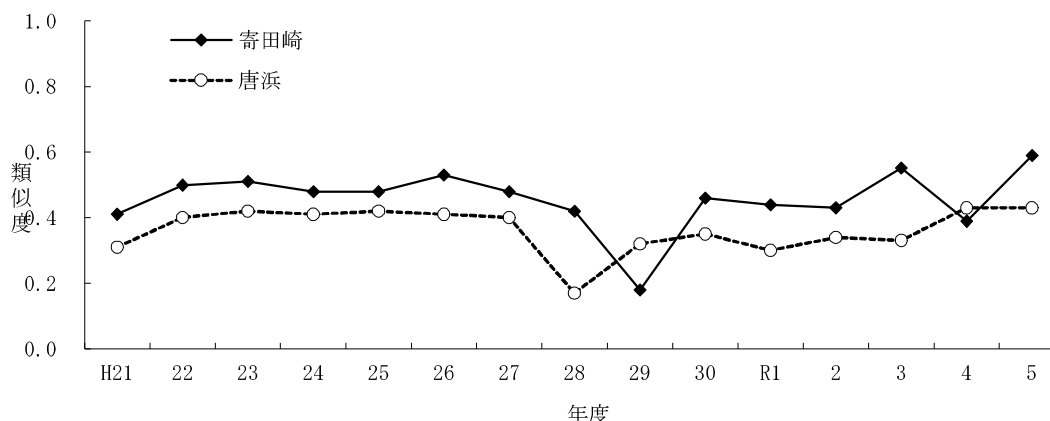
図5 潮間帯生物（動物）の各年度と前年度との年度間類似度
