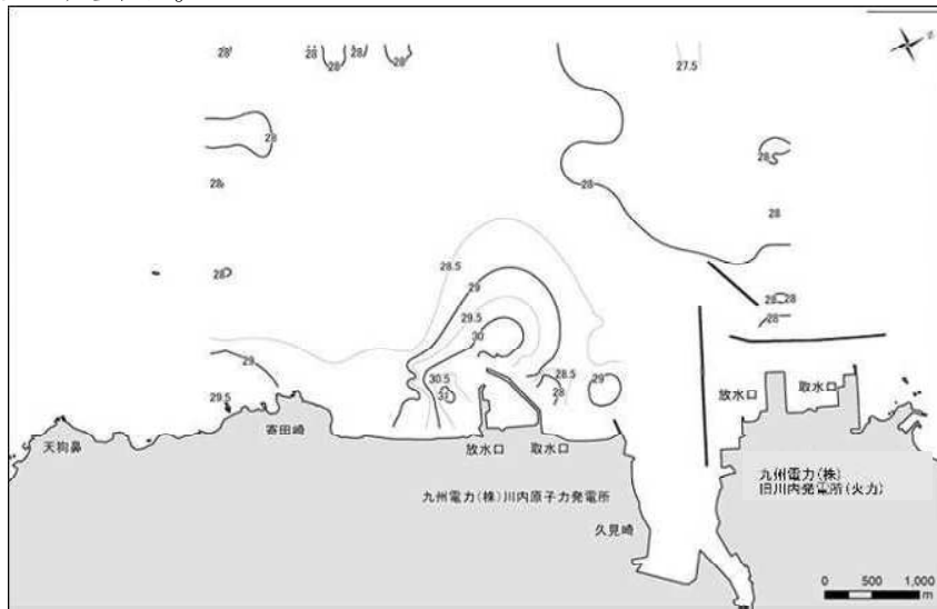
図10-3 2m層水温水平分布 (上げ潮時) 単位:℃
