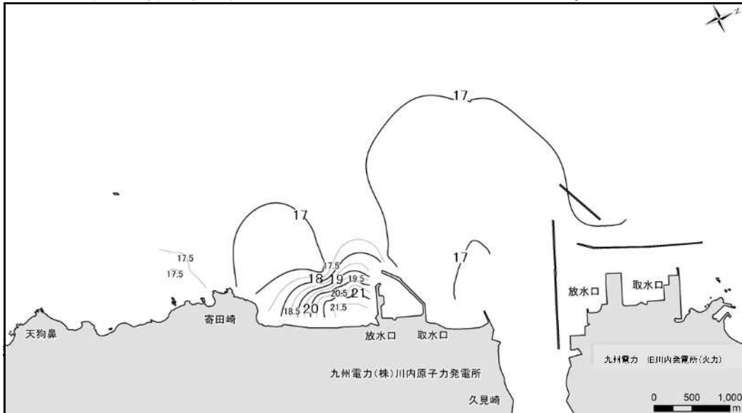
図6-3 2 m層水温水平分布 (上げ潮時) 単位: °C
