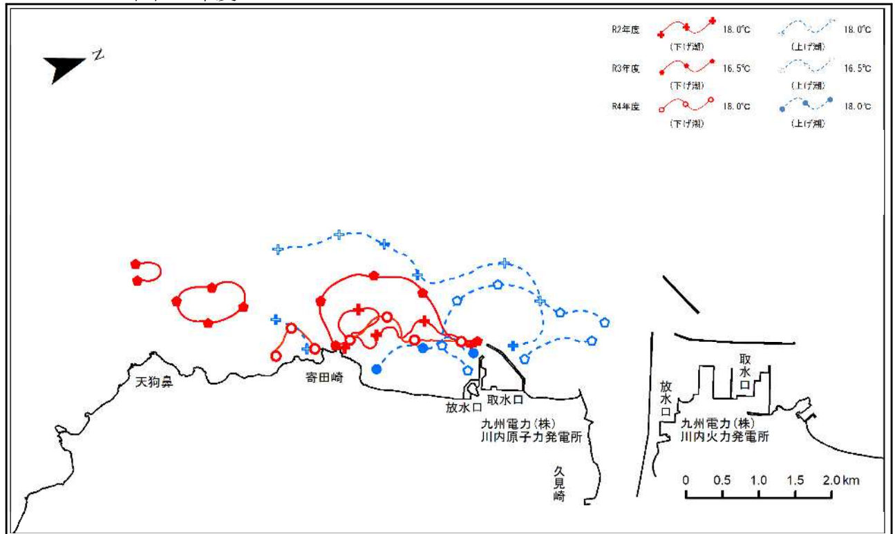
図8-10 令和2年度～4年度冬季表層(0.3m深)温排水拡散範囲
