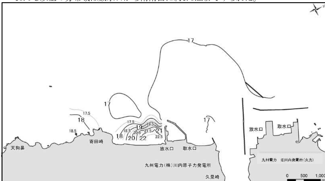
図6-2 1 m層水温水平分布（上げ潮時） 単位：℃
