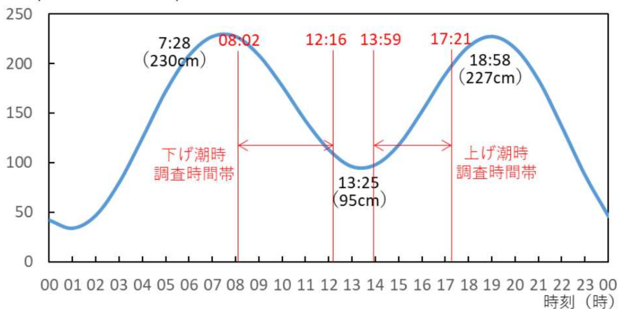
図3 水温・塩分水平分布調査日(令和5年3月5日)の潮汐(阿久根験潮場)と調査時間
