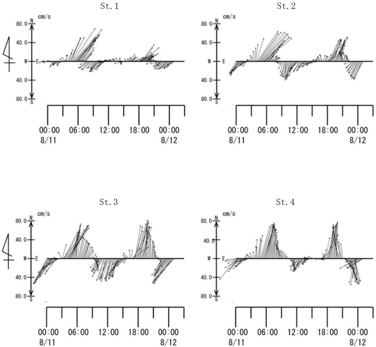
図15-1 25時間調査結果（毎時流ベクトル経時変化）
