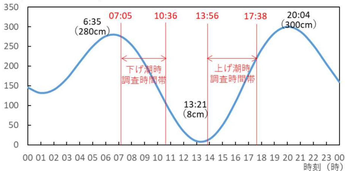
図7 水温・塩分水平分布調査日（令和4年8月11日）の潮汐（阿久根験潮場）と調査時間
