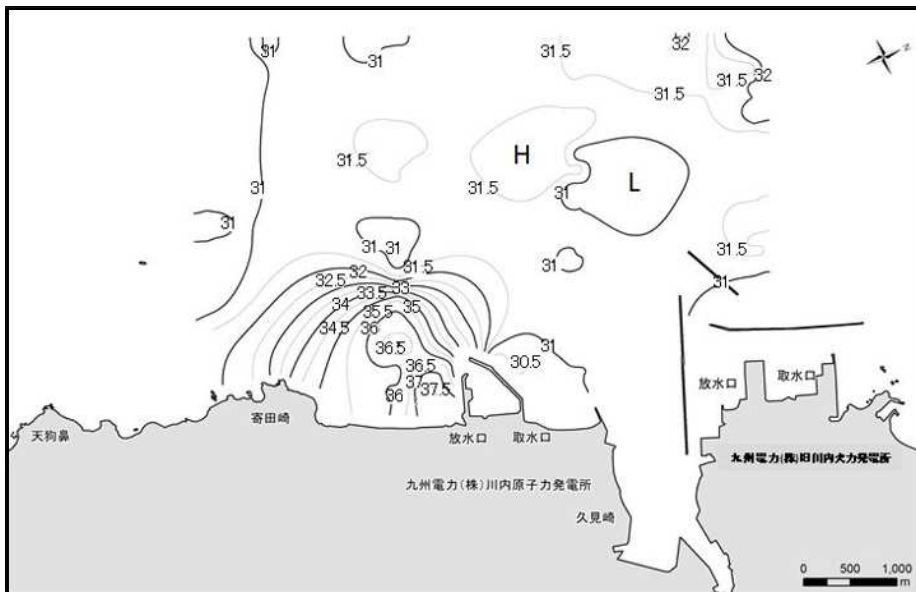
図10-2 1m層水温水平分布（上げ潮時） 単位：℃
