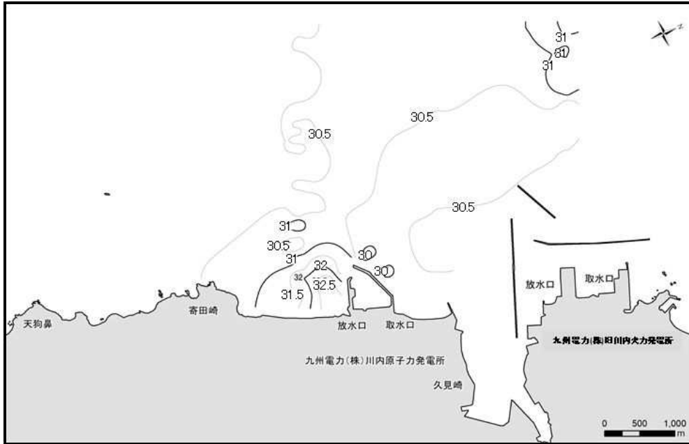
図10-3 2m層水温水平分布（上げ潮時） 単位：℃
