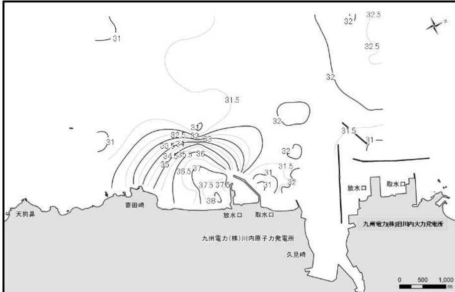
図10-1 表層(0.3m深)水温水平分布（上げ潮時） 単位：℃
