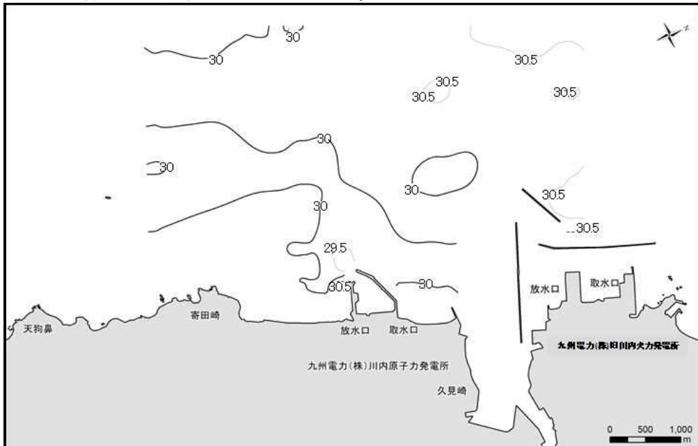
図10-4 3m層水温水平分布（上げ潮時） 単位：℃
