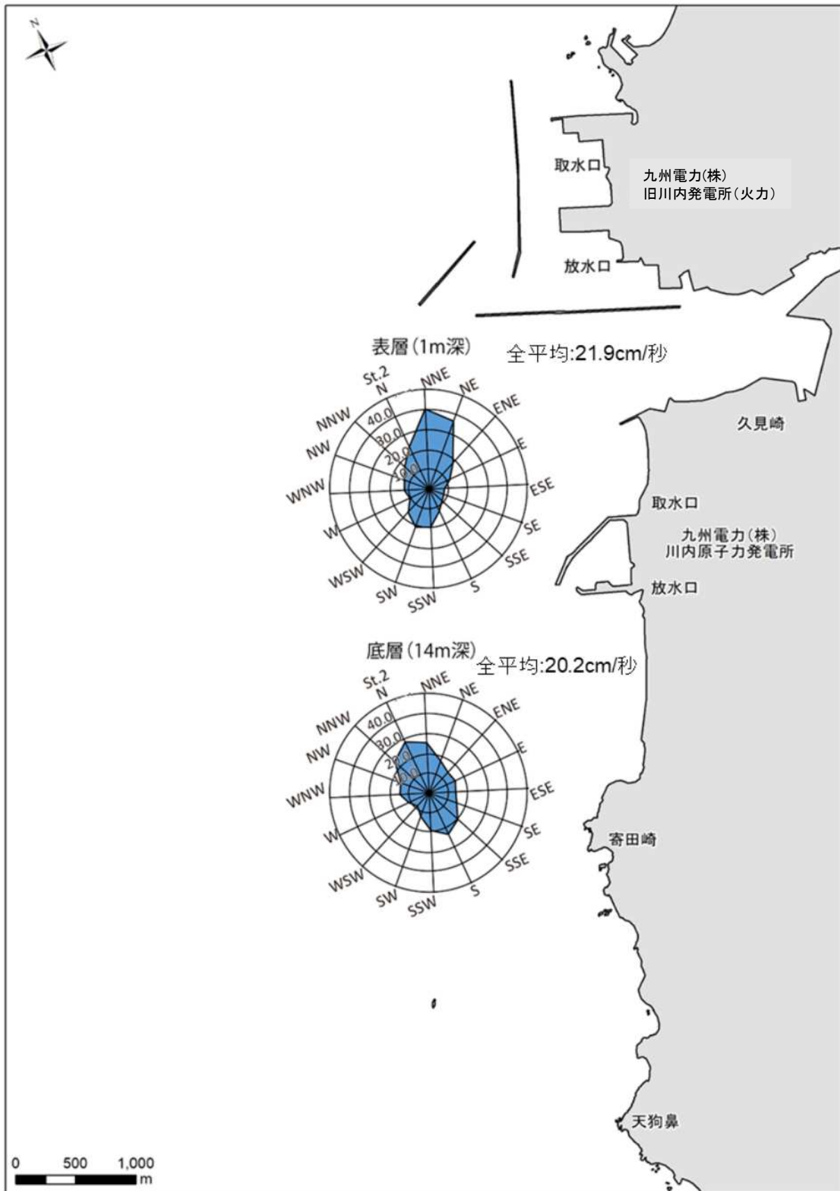
図16-4 15日間調査結果（流向別平均流速分布）
