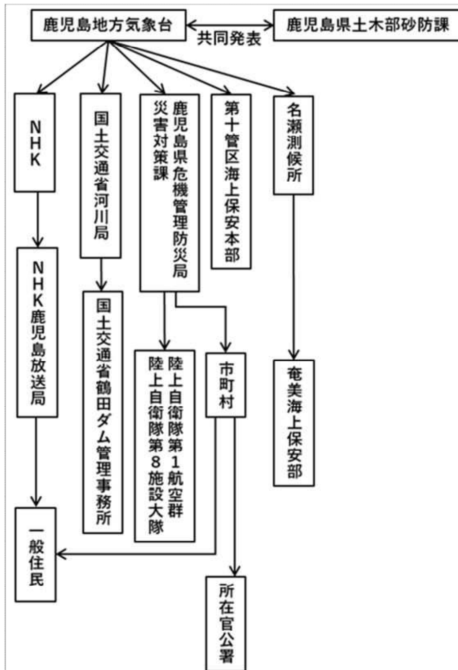
図3. 2. 1. 8 土砂災害警戒情報の伝達系統図（土砂災害警戒情報に関する実施要領による）
