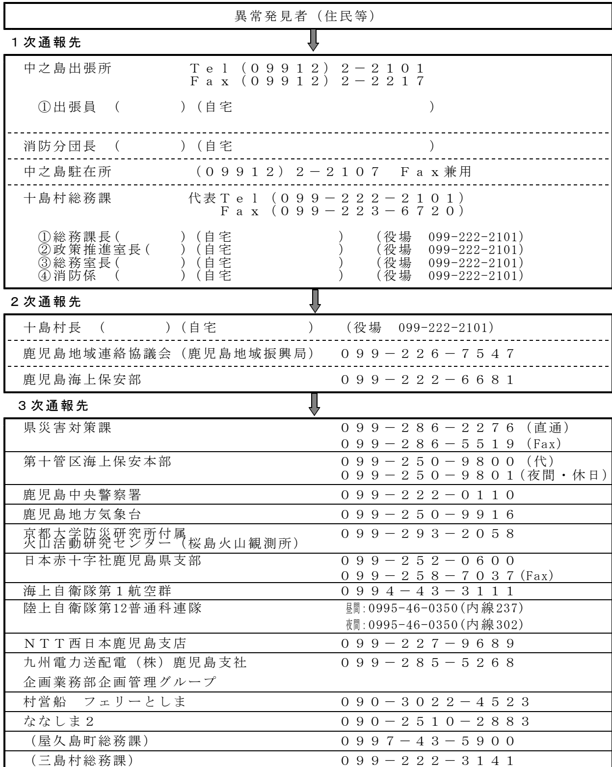
図5-4-4 通報系統
