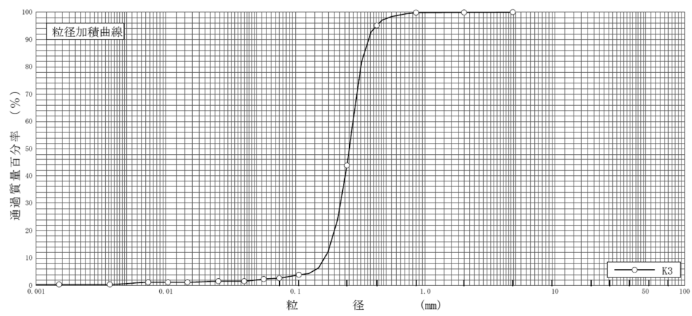
圖 6.6-2(1) 粒徑加積曲線 (秋季)
