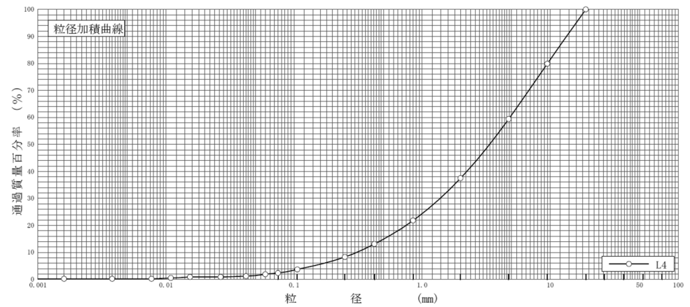
图 6.6-3(1) 粒径加积曲线 (秋季)
