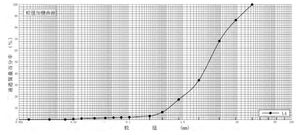
图 6.6-3(3) 粒径加积曲线 (春季)
