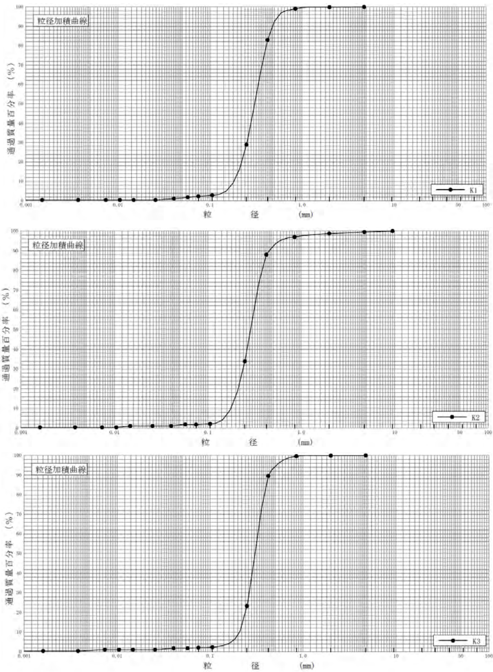
图 6.6-2(4) 粒径加積曲線 (夏季)
