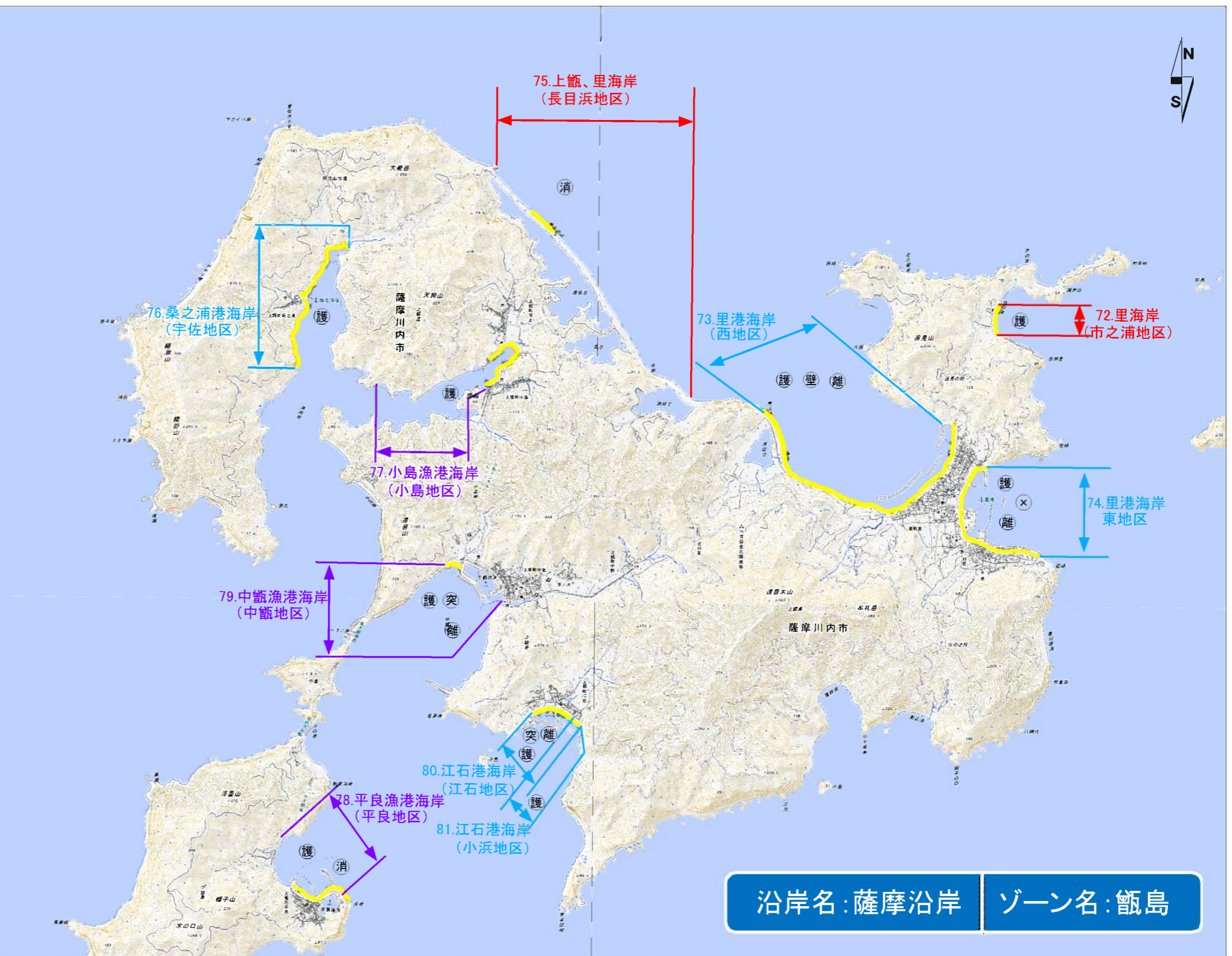
図 海岸保全施設の整備区域、種類、規模及び配置 15/17
