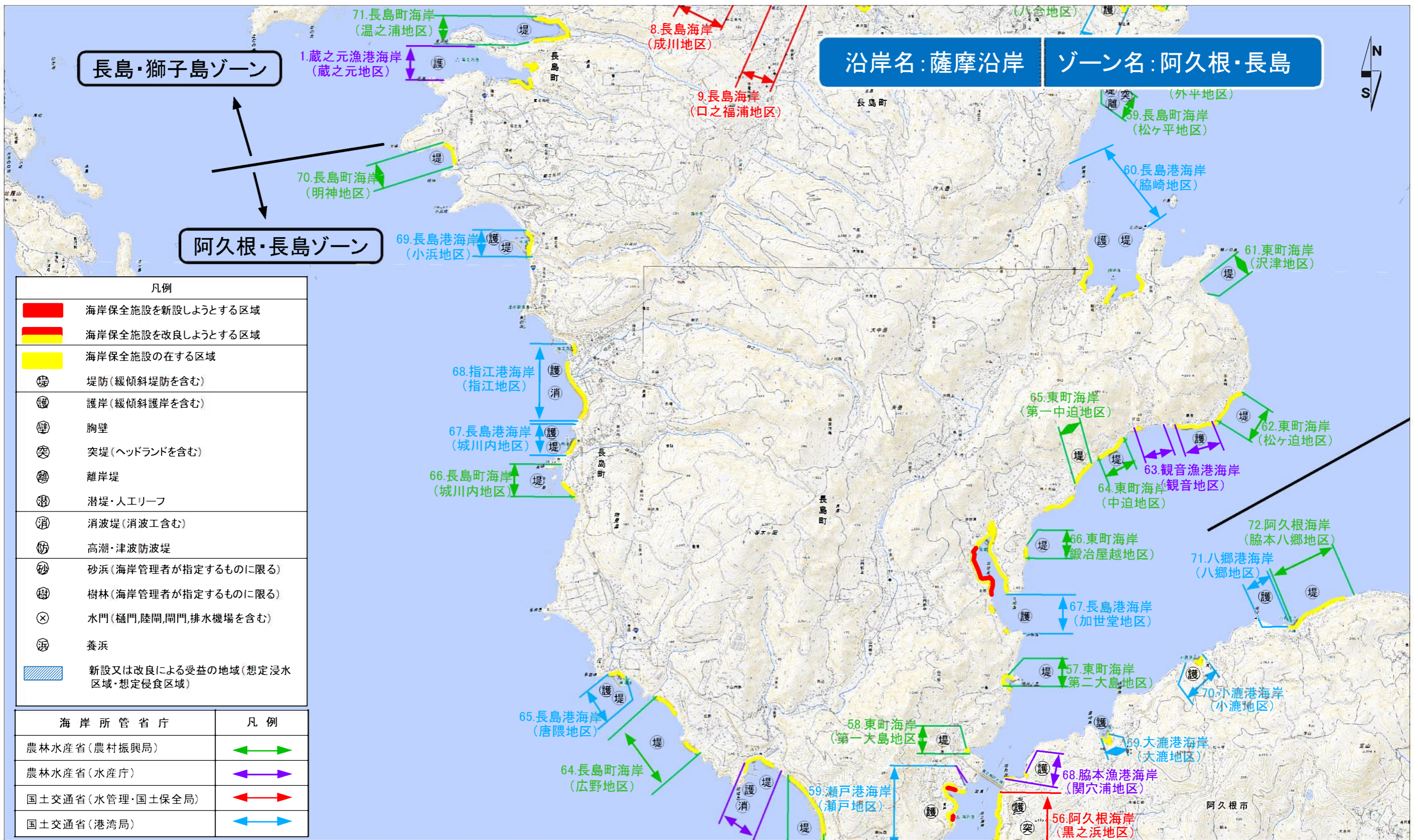
図 海岸保全施設の整備区域、種類、規模及び配置 14/17
