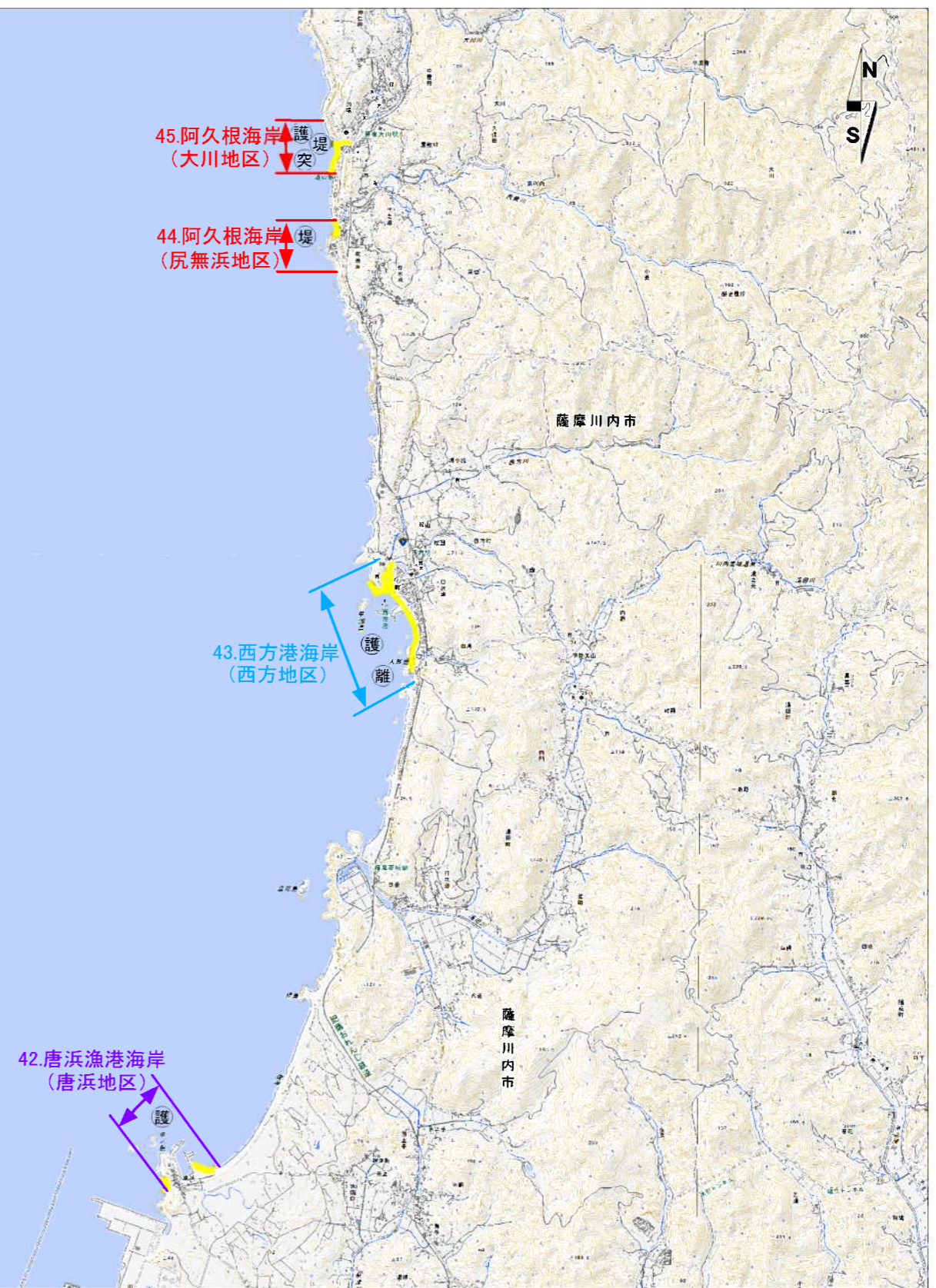
図 海岸保全施設の整備区域、種類、規模及び配置 11/17
