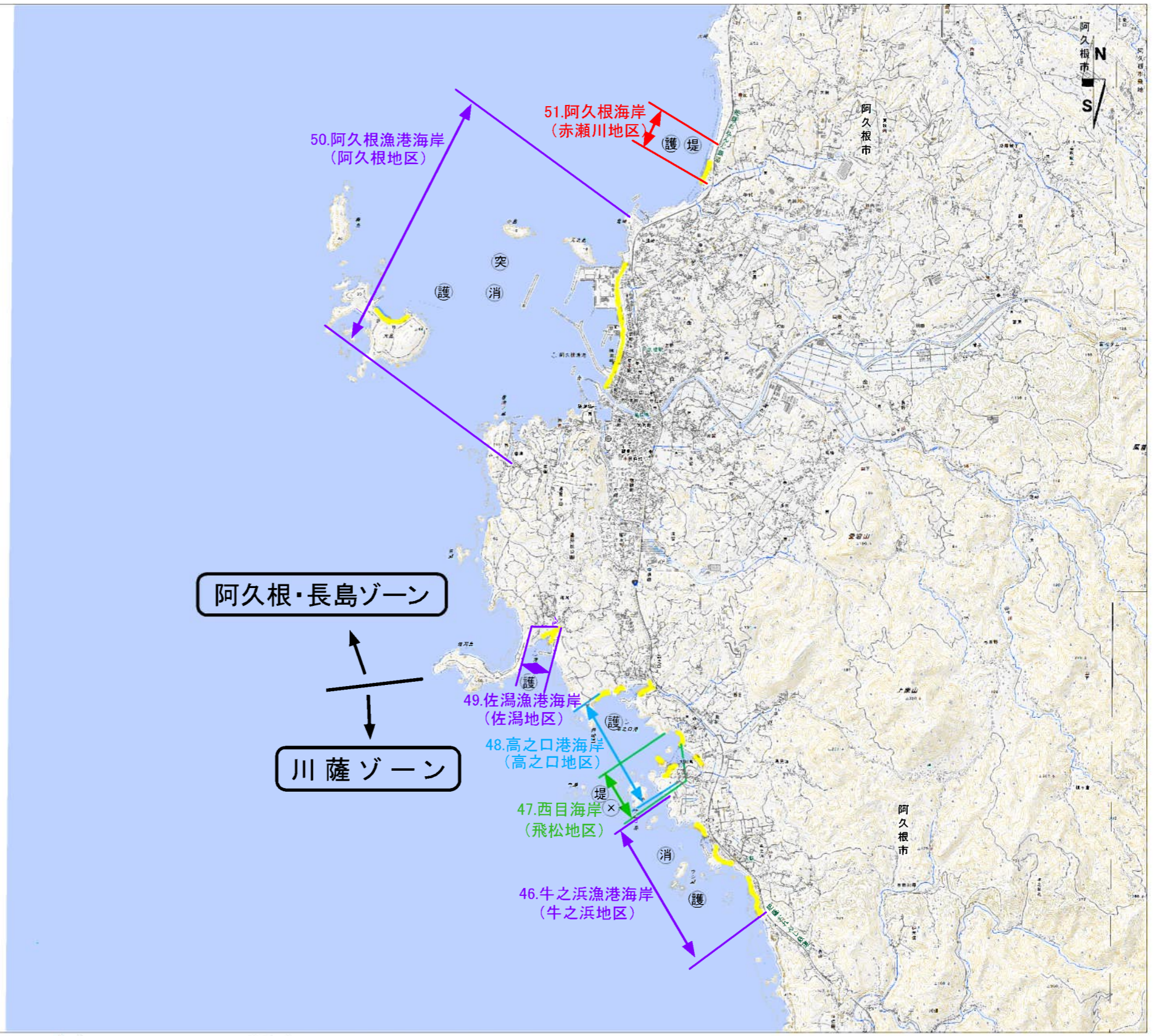
図 海岸保全施設の整備区域、種類、規模及び配置 12/17
