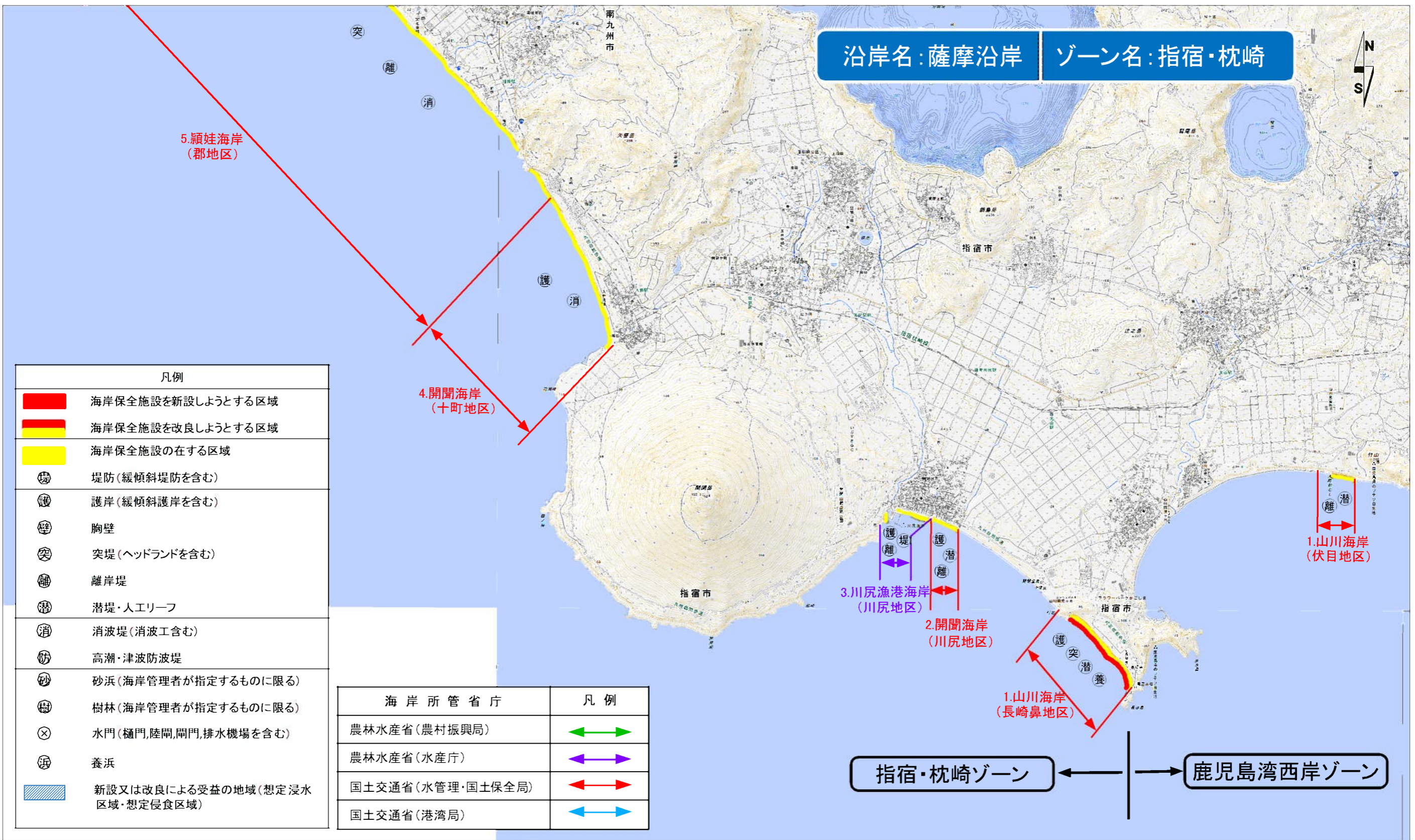
図 海岸保全施設の整備区域、種類、規模及び配置 1/17
