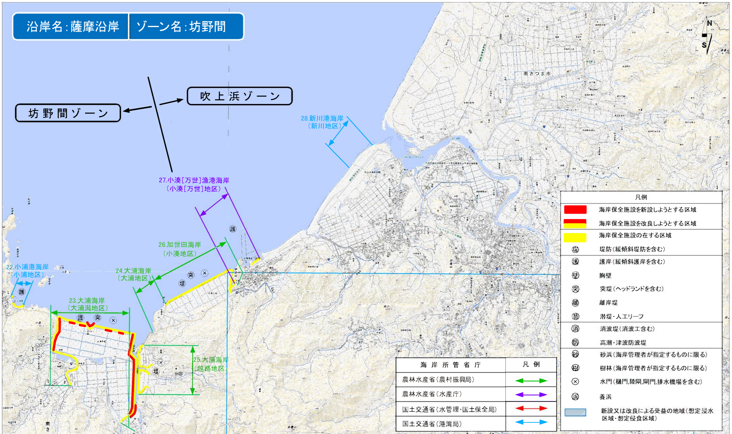
図 海岸保全施設の整備区域、種類、規模及び配置 6/17
