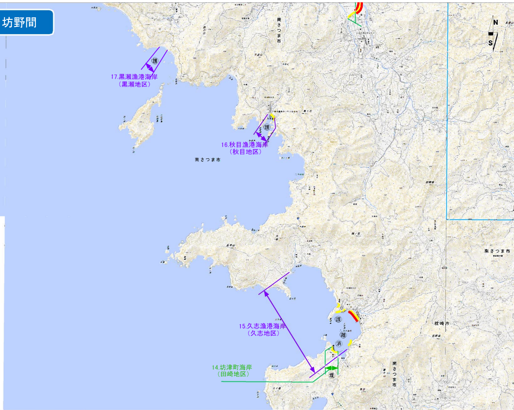
図 海岸保全施設の整備区域、種類、規模及び配置 4/17
