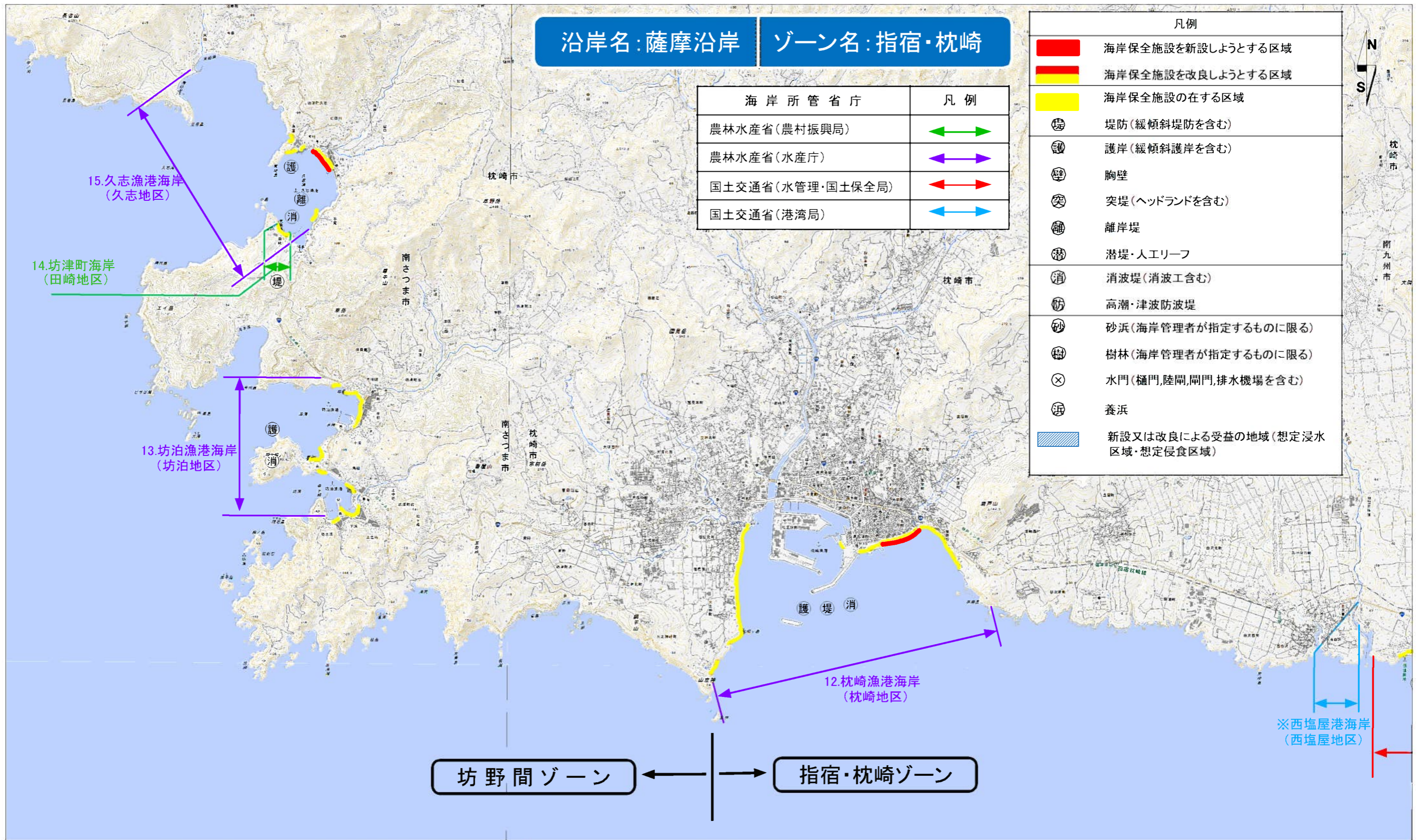
図 海岸保全施設の整備区域、種類、規模及び配置 3/17
