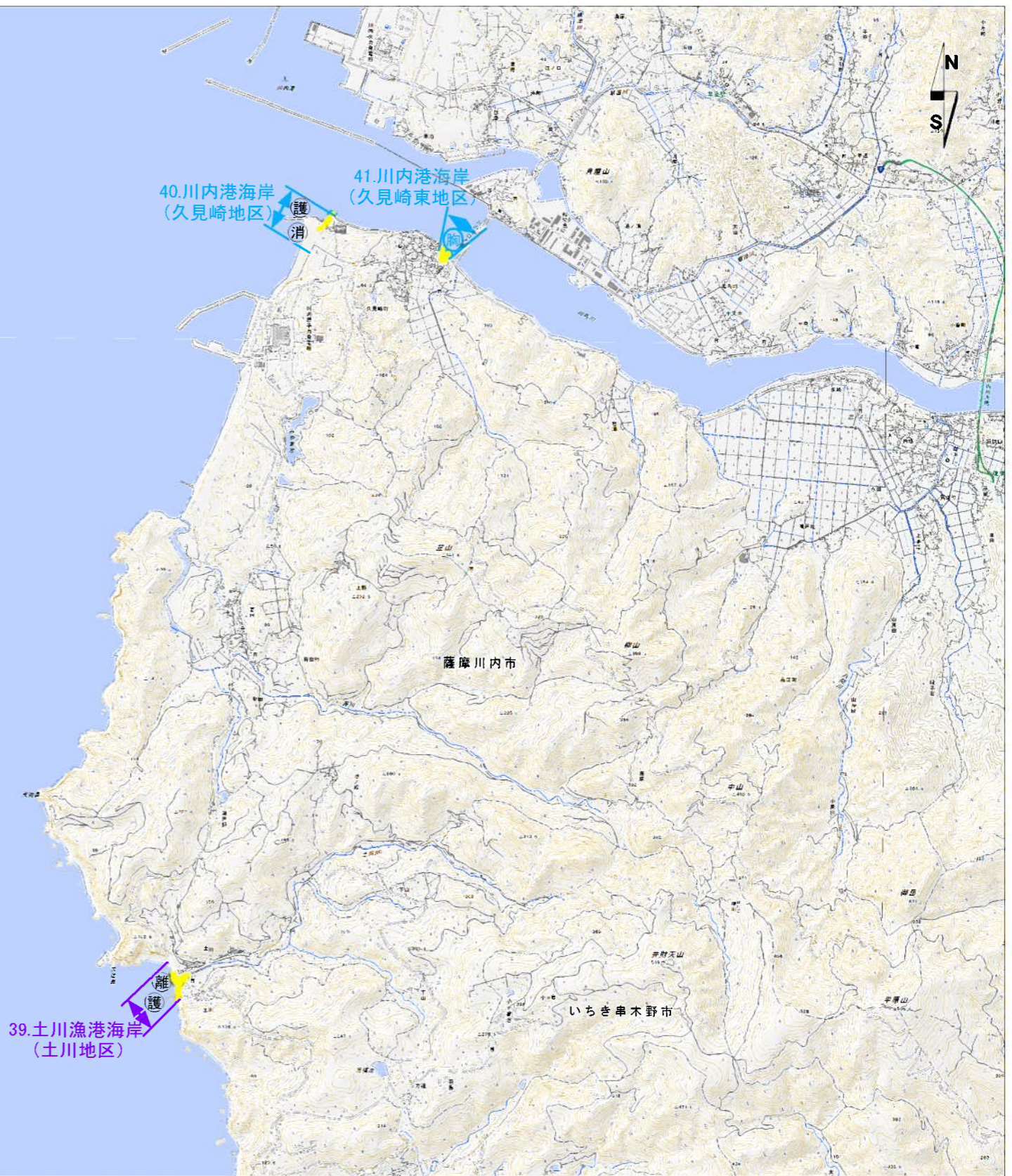
図 海岸保全施設の整備区域、種類、規模及び配置 10/17
