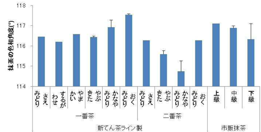
図2 新てん茶ライン製抹茶と市販抹茶の品質比較
