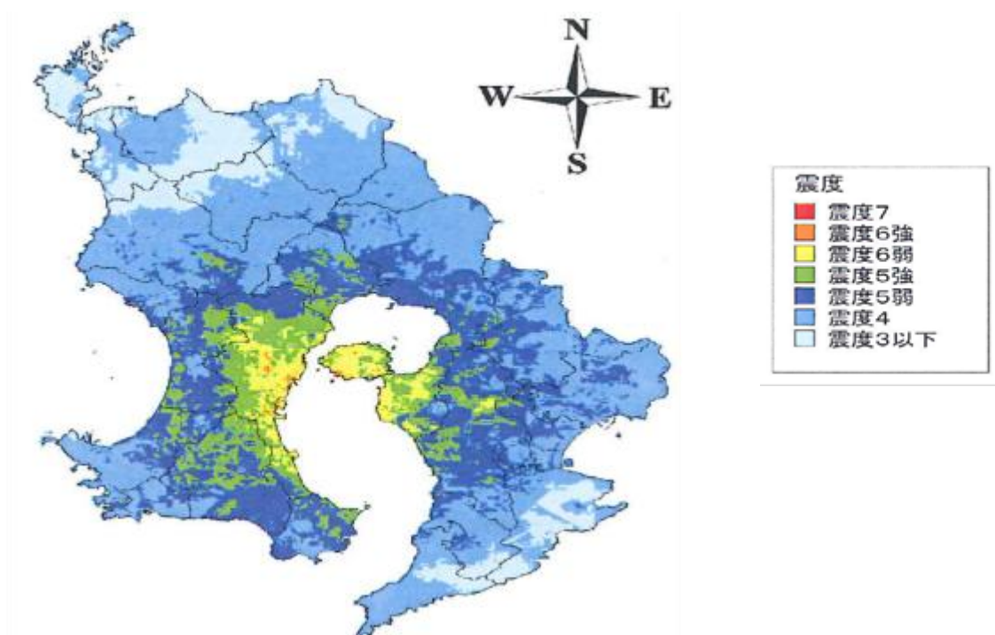
鹿児島湾直下地震の震度分布図
