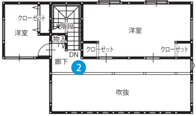
2階平面図
