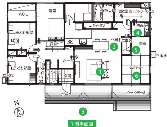
1階平面図
