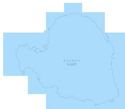
RCP 8.5 2091-2100年
