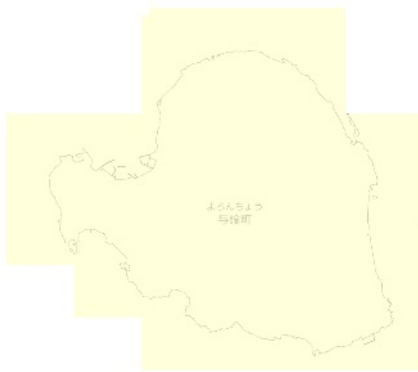
RCP 2.6 21世紀末
