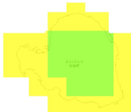
RCP 8.5 2051-2060年
