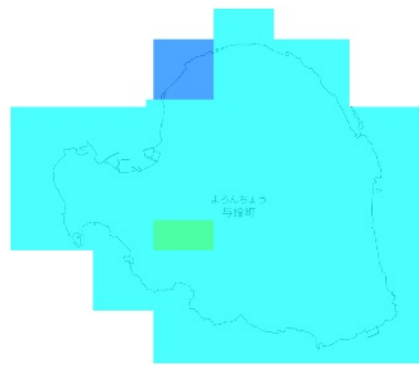
RCP 8.5 2051-2060年
