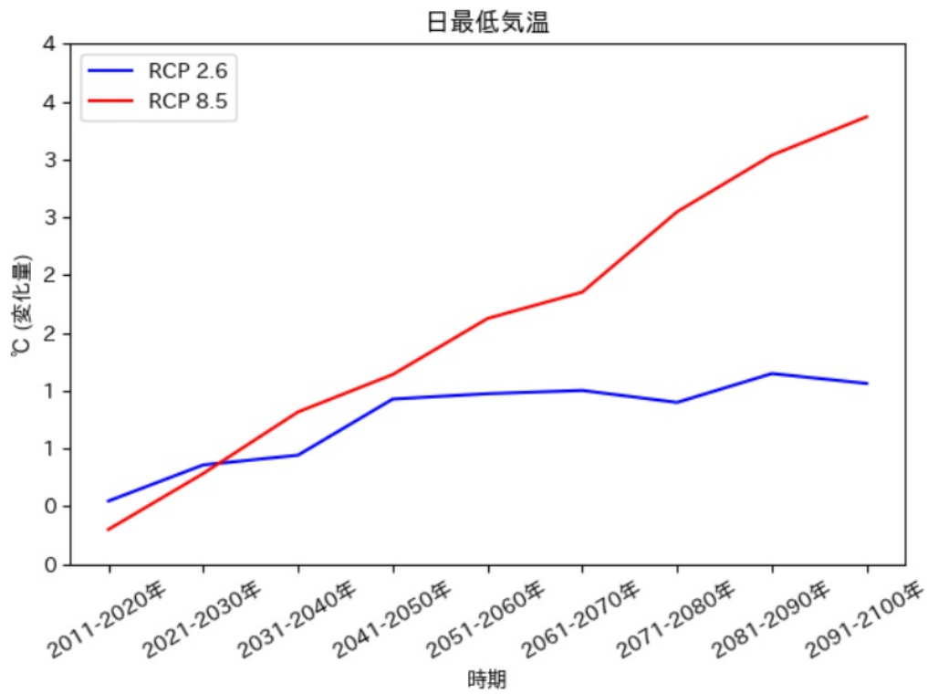
日最低気温の推移予測 (与論町)
