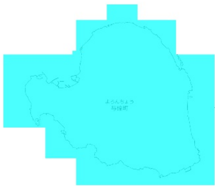
RCP 2.6 2011-2020年
