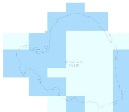
RCP 8.5 2051-2060年
