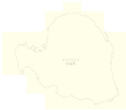
RCP 2.6 2011-2020年
