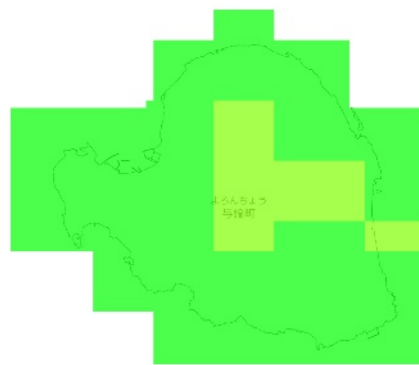
RCP 8.5 2091-2100年
