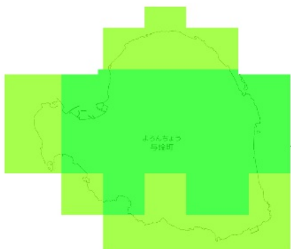
RCP 2.6 2091-2100年
