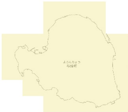
RCP 2.6 21世紀末
