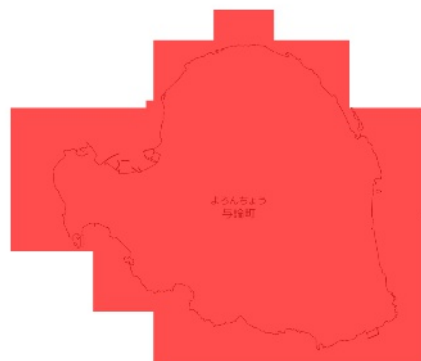
RCP 8.5 2091-2100年
