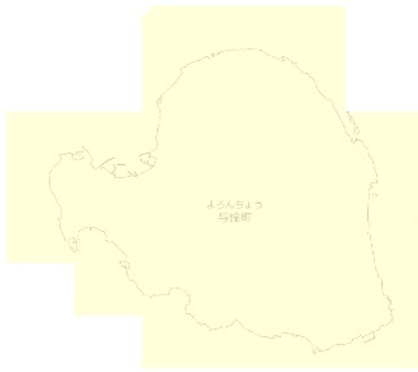
RCP 2.6 21世紀半ば
