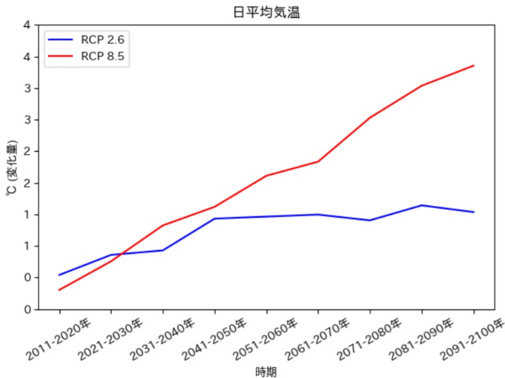
日平均気温の推移予測 (与論町)
