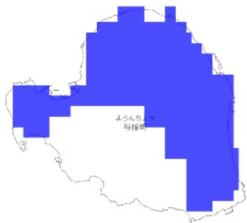
RCP 2.6 2081-2100年
