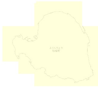
RCP 8.5 21世紀半ば
