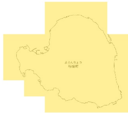
RCP 8.5 21世紀末
