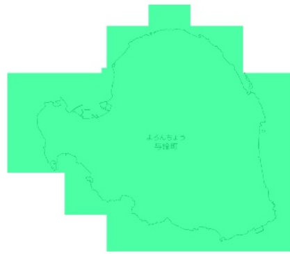
RCP 8.5 2011-2020年
