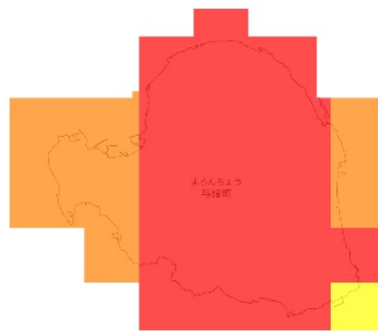
RCP 8.5 2091-2100年
