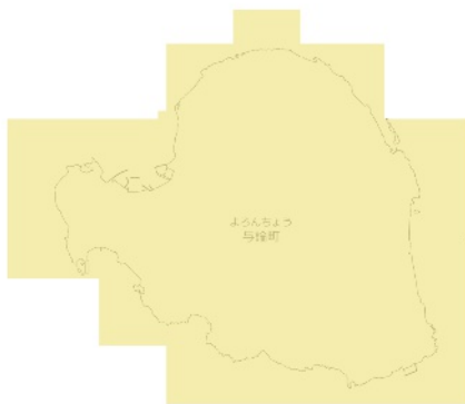
RCP 2.6 2051-2060年
