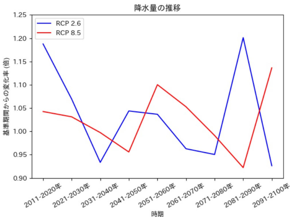
降水量の推移予測 (与論町)
