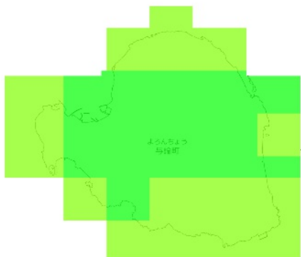
RCP 2.6 2051-2060年
