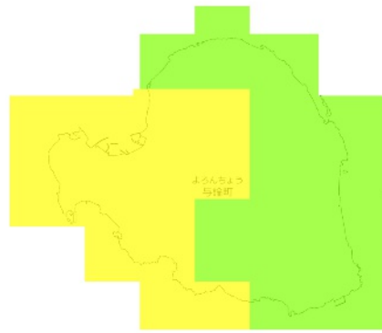
RCP 8.5 2011-2020年
