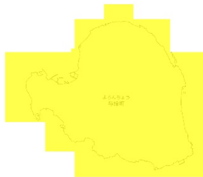
RCP 8.5 2051-2060年
