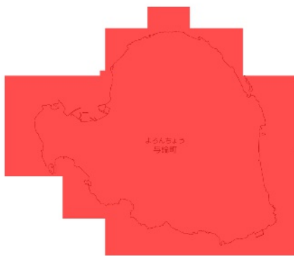
RCP 2.6 2091-2100年
