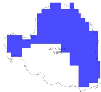
RCP 8.5 2081-2100年
