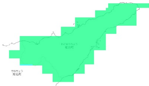
RCP 2.6 2051-2060年
