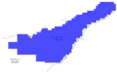
RCP 8.5 2081-2100年
