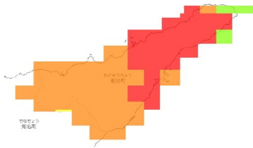
RCP 2.6 2091-2100年
