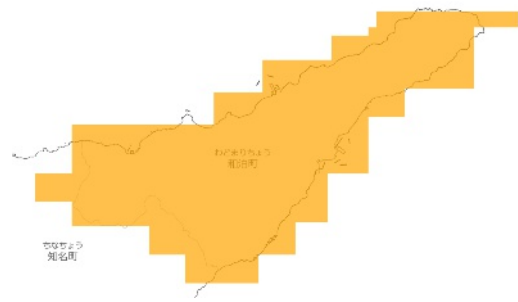
RCP 8.5 2091-2100年
