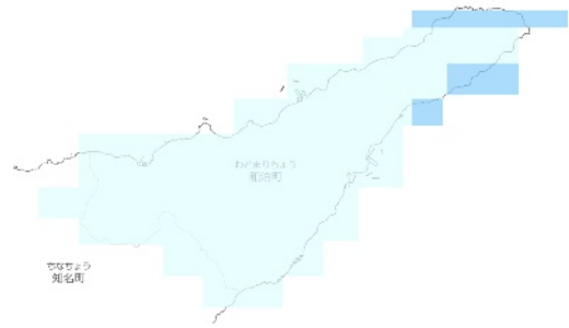
RCP 8.5 2051-2060年
