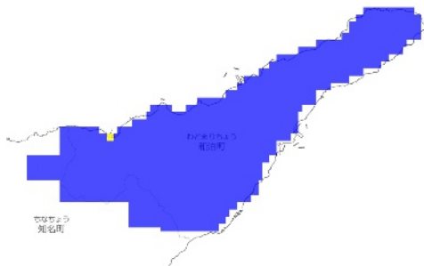
RCP 2.6 2081-2100年
