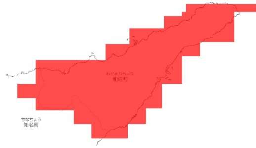
RCP 8.5 2091-2100年
