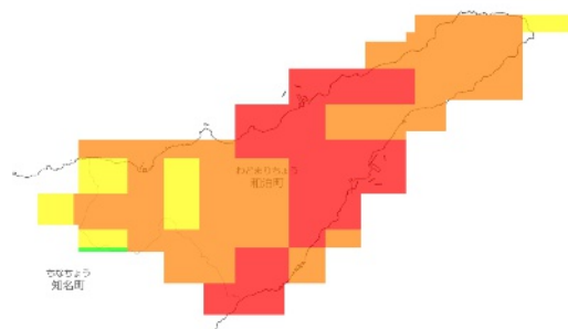
RCP 8.5 2091-2100年
