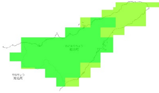
RCP 2.6 2051-2060年
