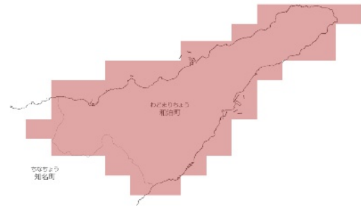
RCP 8.5 21世紀末
