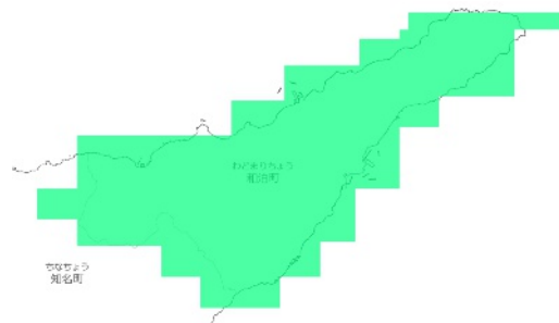
RCP 8.5 2051-2060年
