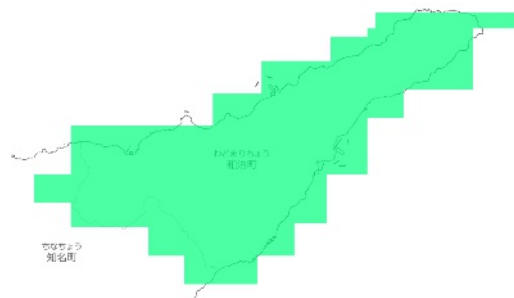
RCP 8.5 2011-2020年
