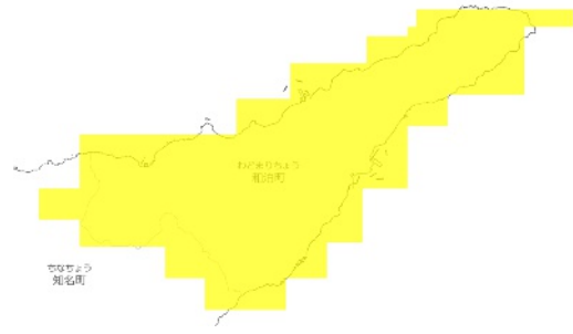
RCP 8.5 2051-2060年
