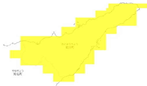
RCP 8.5 2051-2060年
