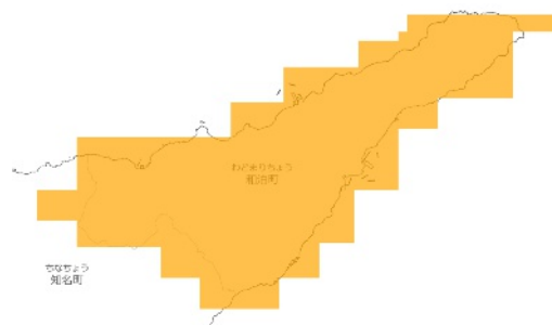
RCP 8.5 2091-2100年
