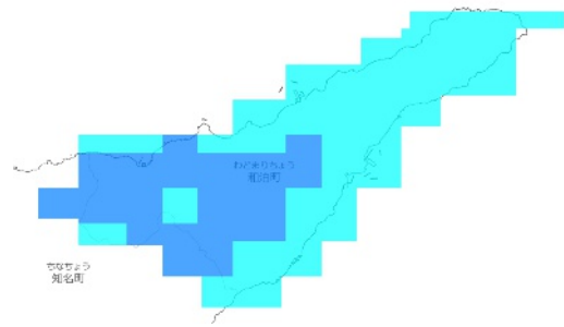
RCP 8.5 2011-2020年
