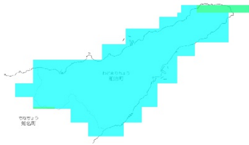
RCP 2.6 2011-2020年
