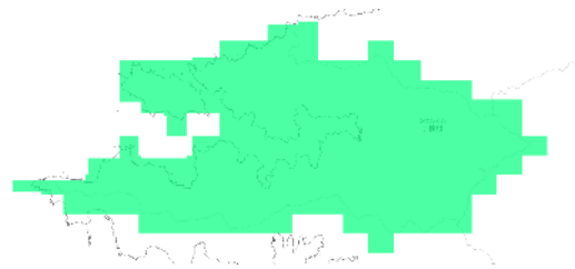
RCP 8.5 2011-2020年
