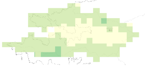
RCP 2.6 21世紀末
