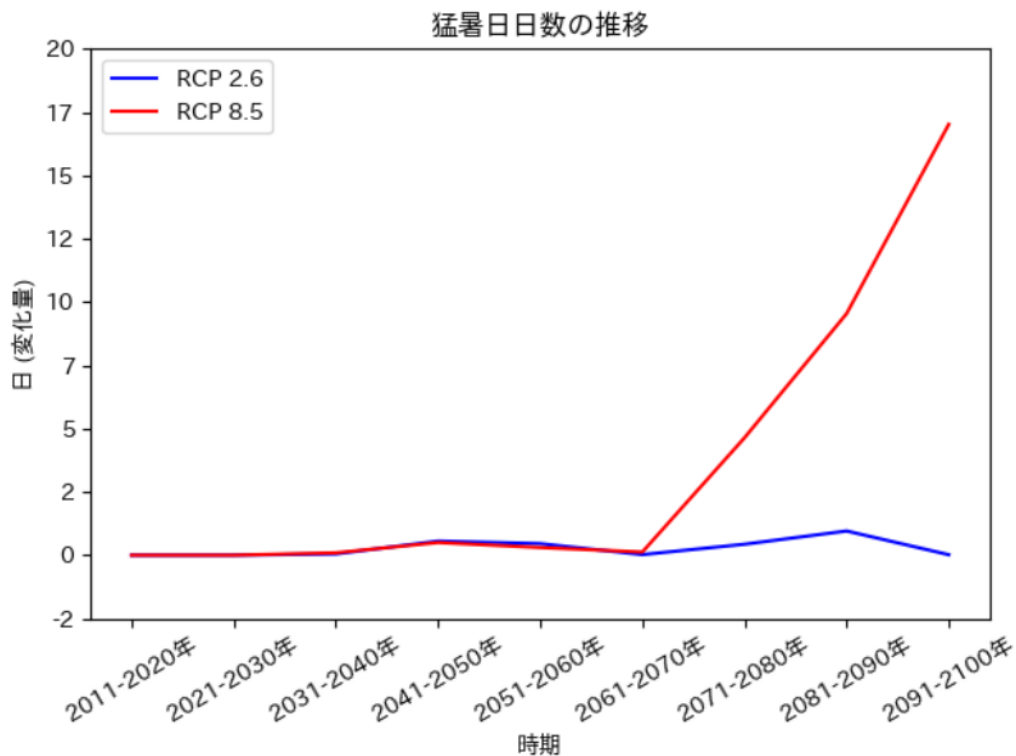
猛暑日の推移予測 (宇検村)
