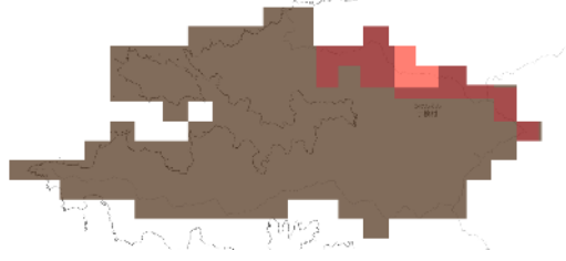
RCP 2.6 21世紀末
