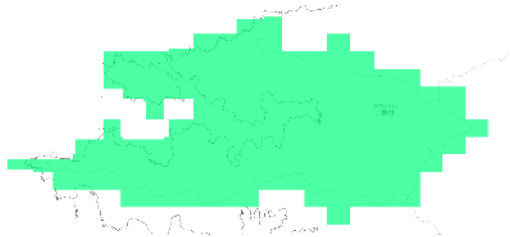
RCP 2.6 2091-2100年
