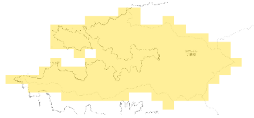
RCP 8.5 21世紀末
