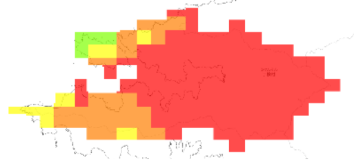
RCP 8.5 2091-2100年
