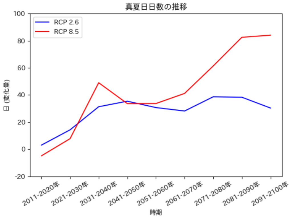
真夏日の推移予測 (宇検村)
