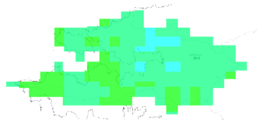
RCP 8.5 2011-2020年
