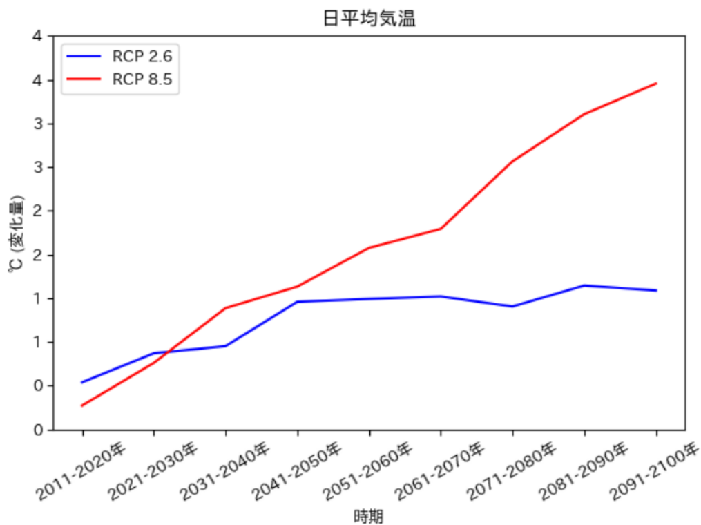
日平均気温の推移予測 (宇検村)
