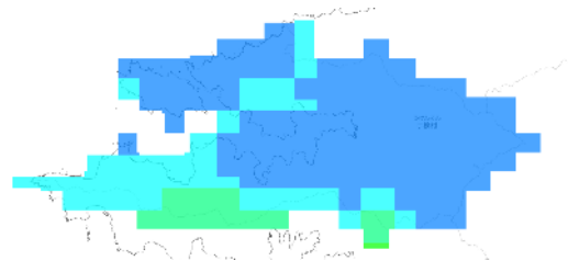
RCP 8.5 2011-2020年
