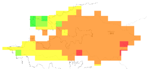
RCP 2.6 2011-2020年
