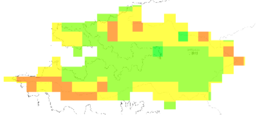
RCP 2.6 2051-2060年
