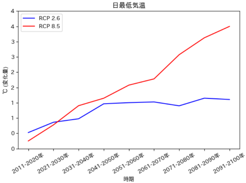
日最低気温の推移予測 (宇検村)
