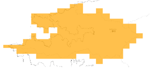
RCP 8.5 2091-2100年
