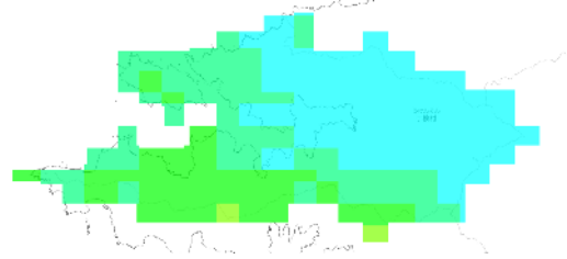
RCP 8.5 2091-2100年
