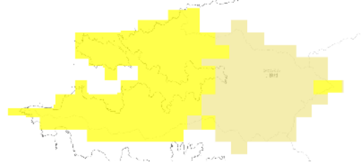
RCP 8.5 2051-2060年
