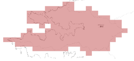
RCP 8.5 21世紀末
