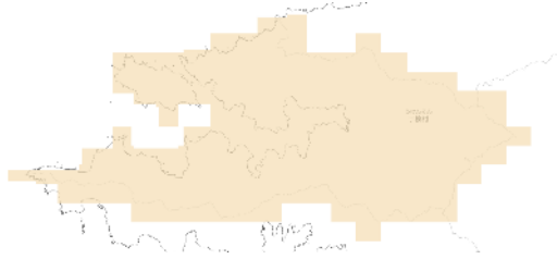
RCP 2.6 2091-2100年
