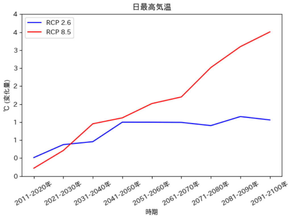
日最高気温の推移予測 (宇検村)
