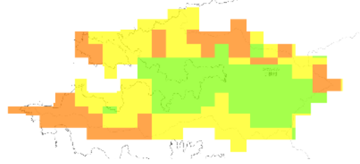
RCP 8.5 2051-2060年
