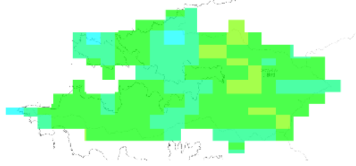
RCP 2.6 2051-2060年
