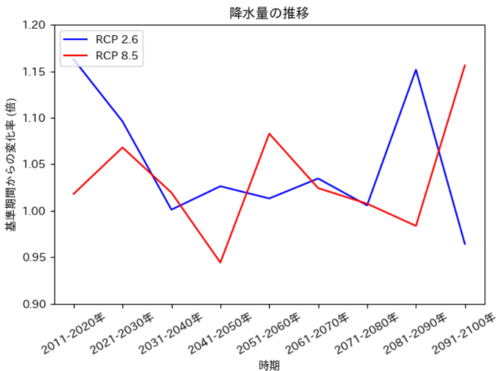
降水量の推移予測 (宇検村)
