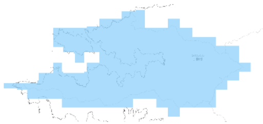
RCP 2.6 2011-2020年
