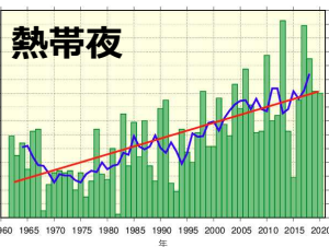
緑の棒：各年の猛暑日・熱帯夜の年間日数 青の太線：猛暑日・熱帯夜の年間日数の5年移動平均 赤の直線：この期間の長期変化傾向
