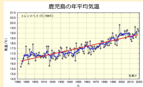
黒の細線：年平均気温 青の太線：気温の5年移動平均 赤の直線：この期間の長期変化傾向 * 地球温暖化に加え都市化や自然変動も含む
