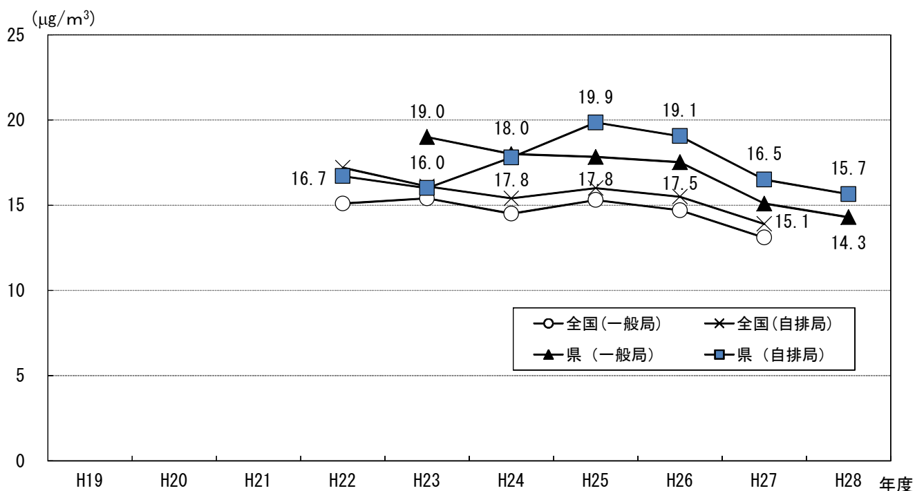
図6 微小粒子状物質（PM2.5）の年平均値の推移
