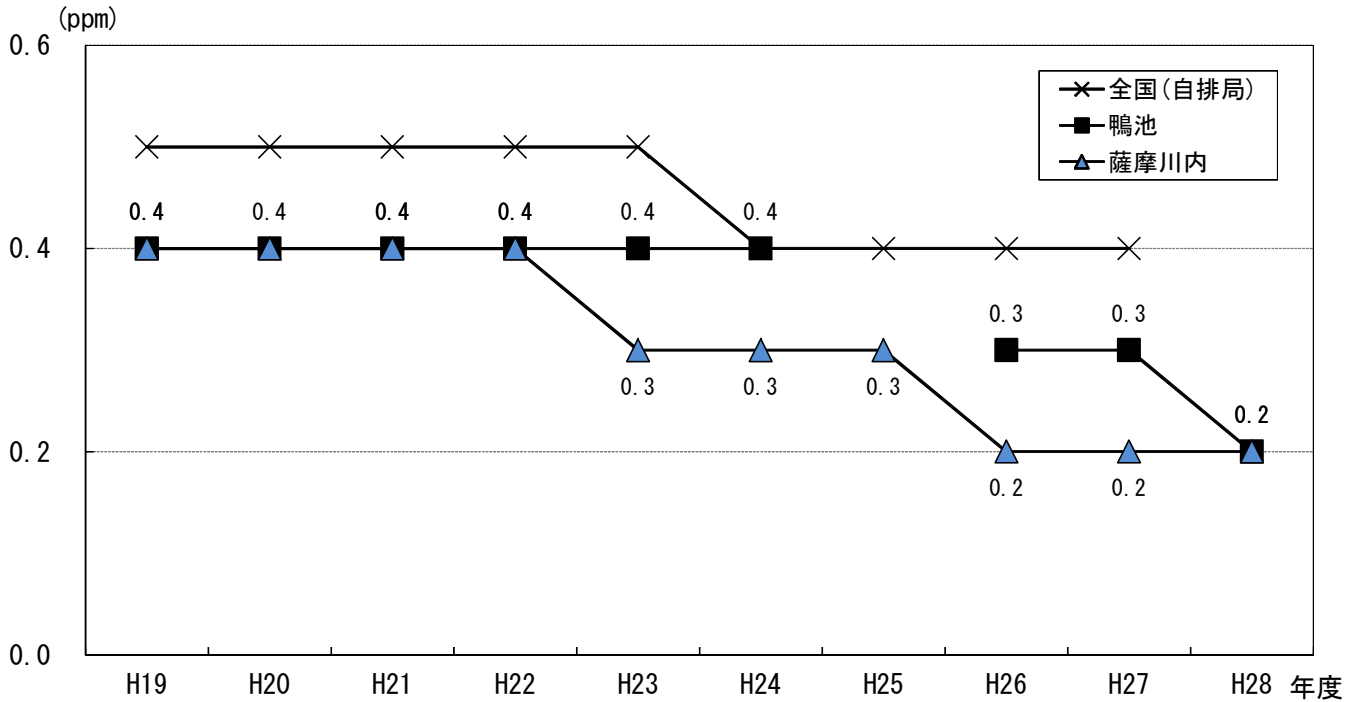
図5 一酸化炭素（CO）の年平均値の推移
