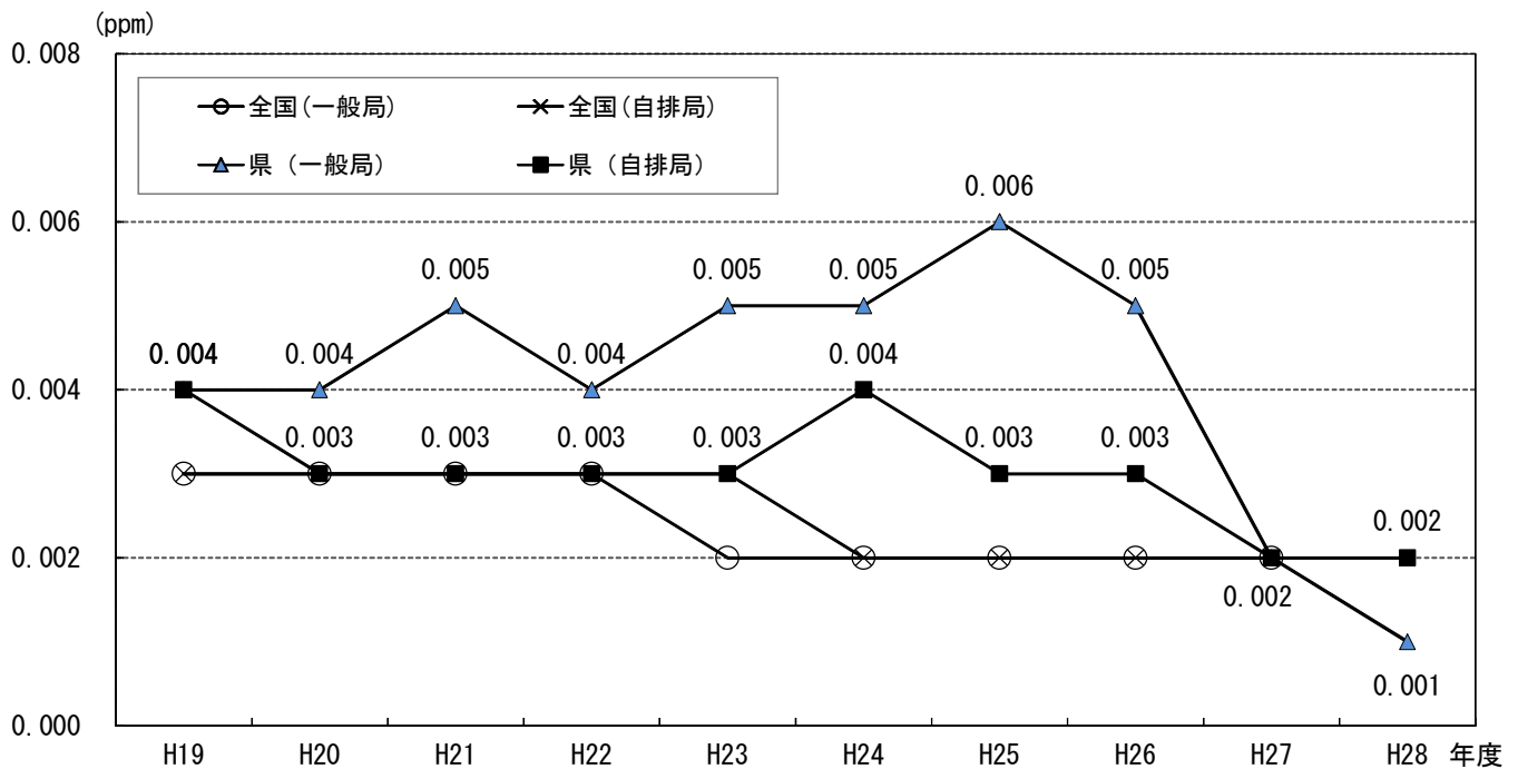
図1 二酸化硫黄（SO 2 ）の年平均値の推移
