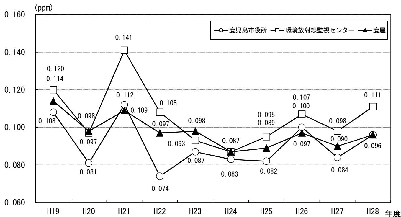
図4 光化学オキシダント（Ox）の昼間の1時間値の最高値の推移
