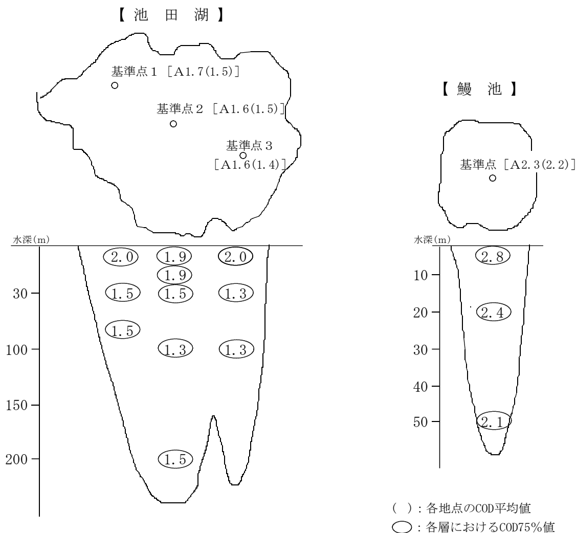
図-5 県内公共用水域の水質現況（湖沼：COD）
