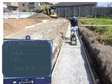
基礎材
