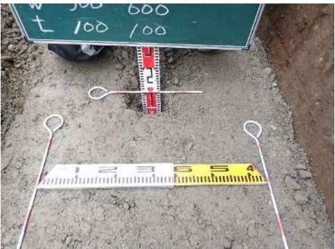
基礎材
