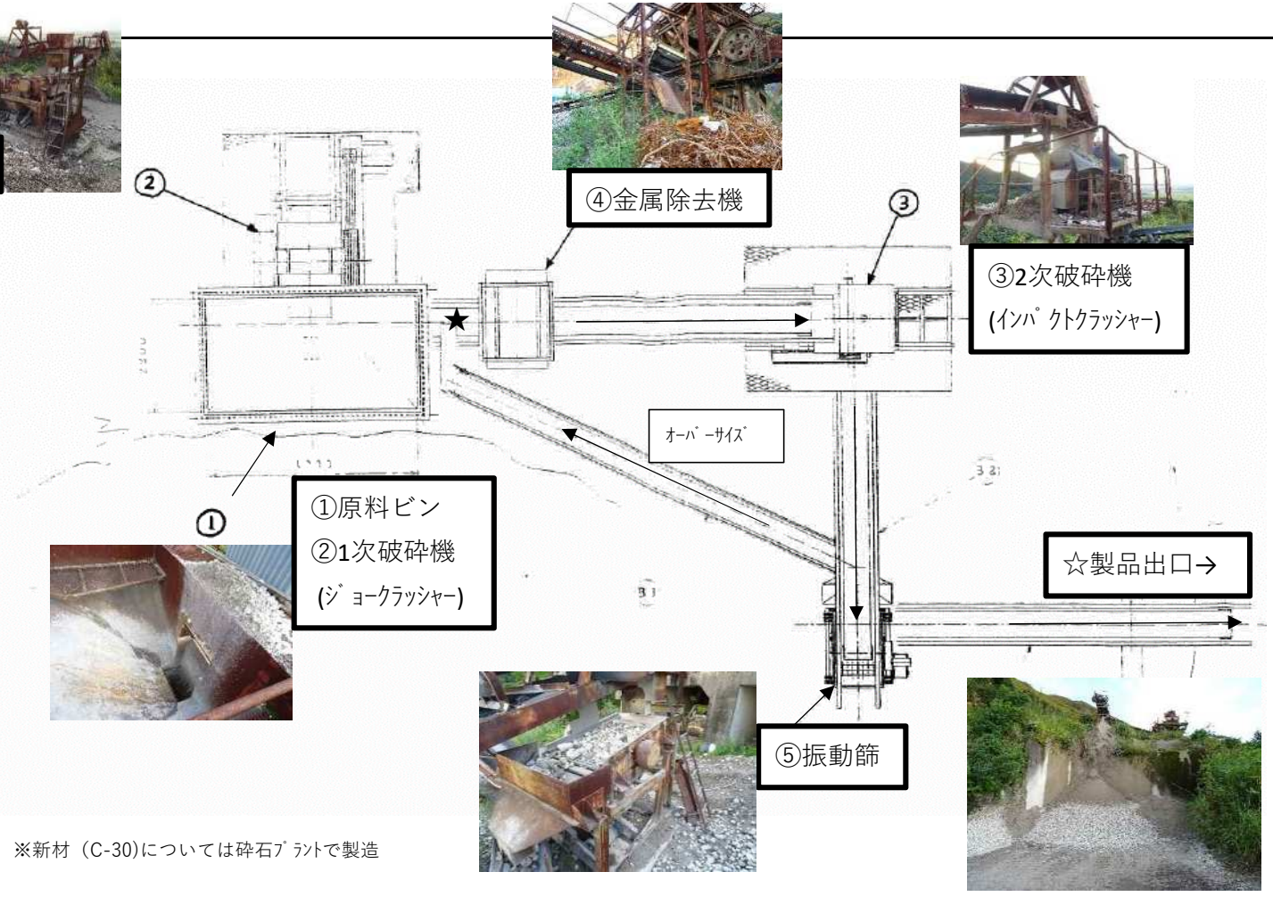
プラント全景
