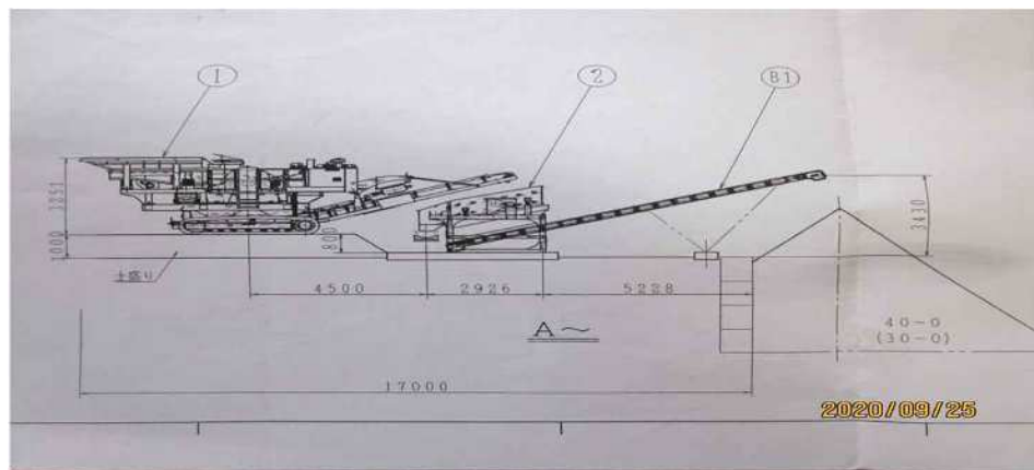
全体図面 中山鉄工所 ジョークラッシャー NC320 GXC 振動型ふるい機 NREH 382 A
