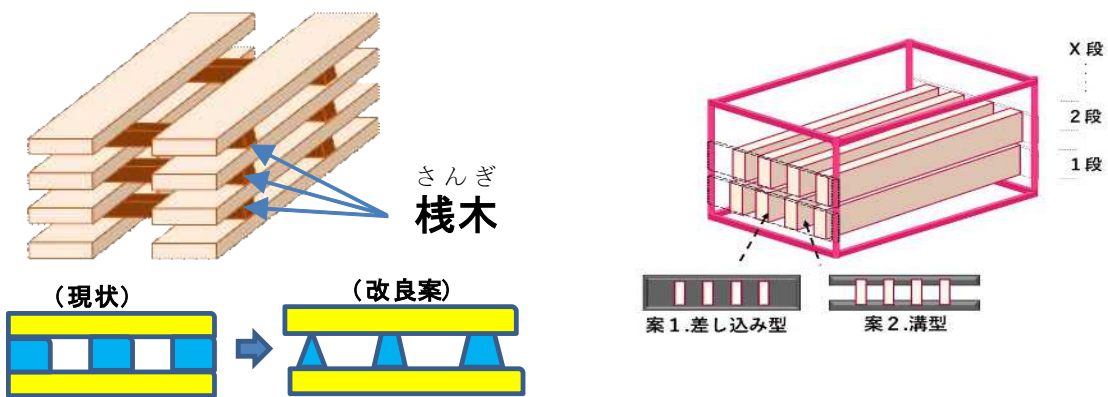
さんぎ 栈木形状の工夫
