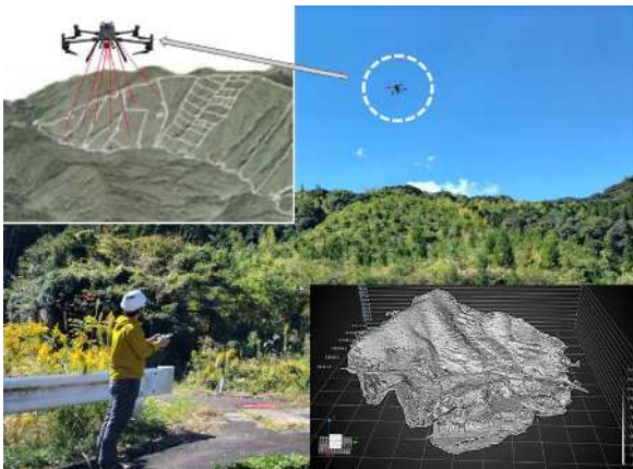
ドローンレーザ計測による地形解析 (森林管理イノベーション導入事業)
