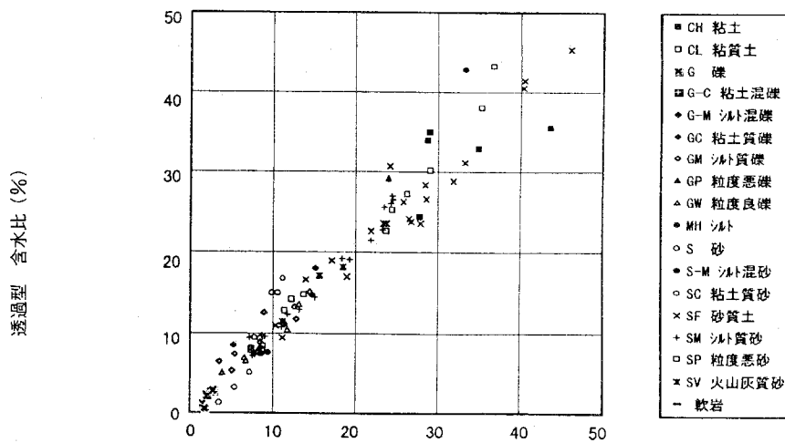
図-8 砂置換と透過型の相関 (含水比・土質別データ)
