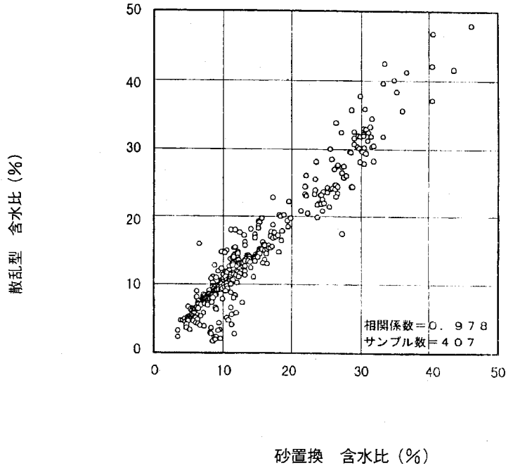
図-3 砂置換と散乱型の相関 (含水比・全データ)
