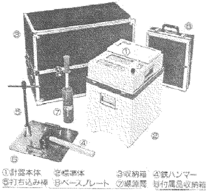
図-4 計器の構成例（透過型）
