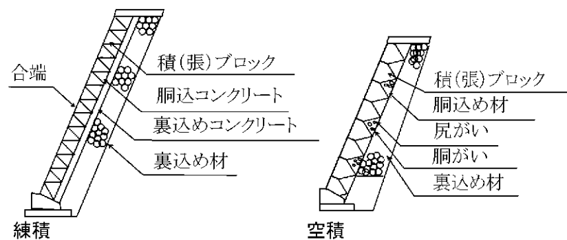
図3-2-5 コンクリートブロック工
