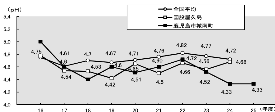
図3-10 年平均値(pH)の推移
