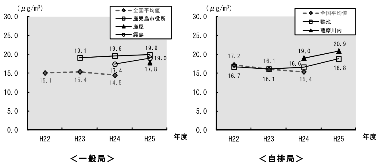
図3-9 微小粒子状物質の年平均値の推移
