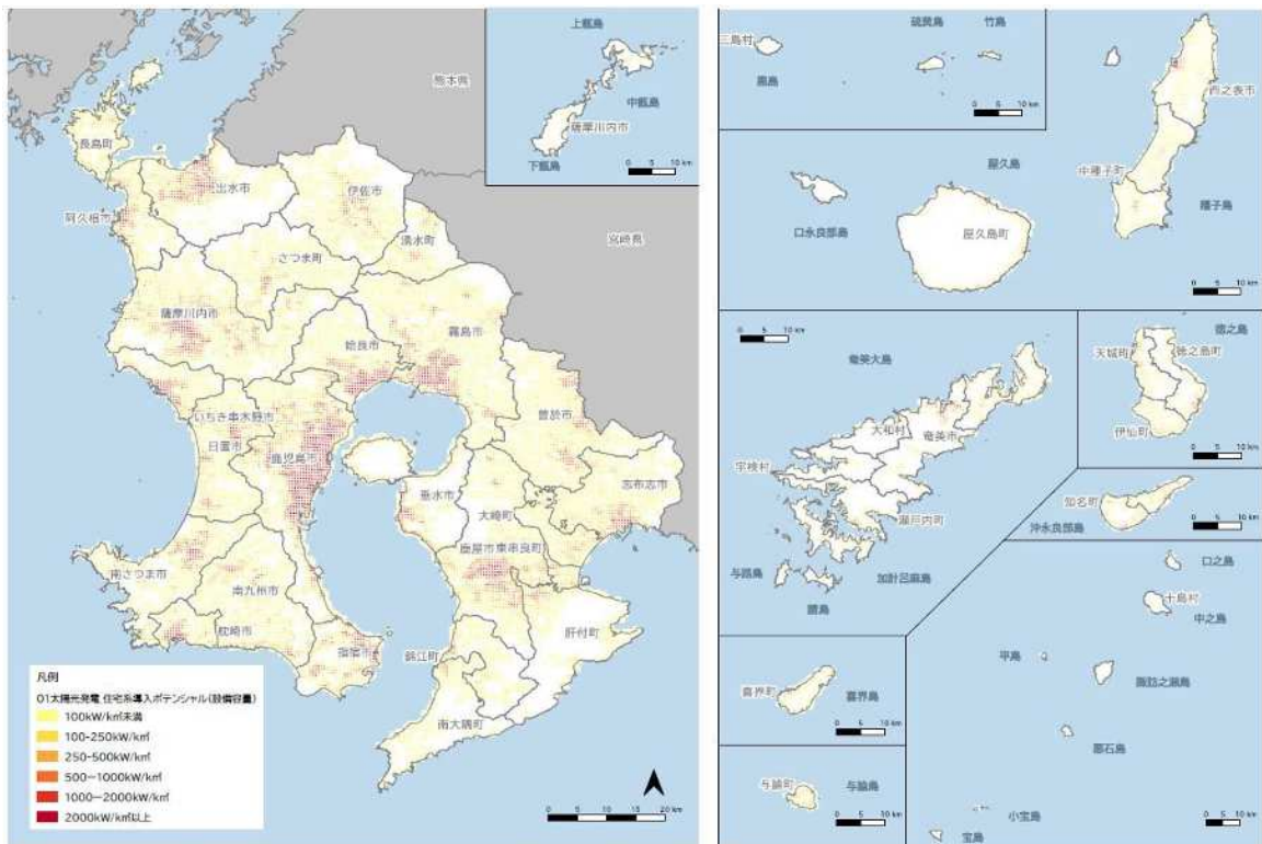
図 4-3 太陽光発電導入ポテンシャル
