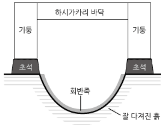
▲하시가카리 하부 구조
