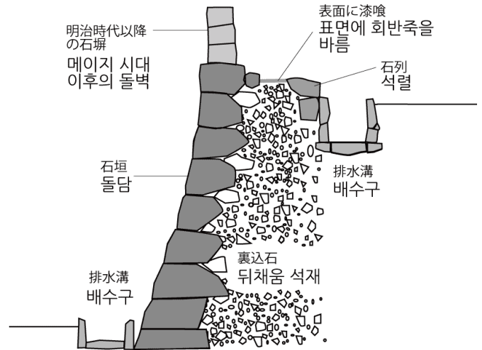
▲ 돌담과 배수구 모식도
